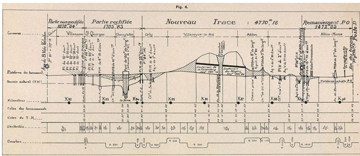
Voie ferrée dit raccordement de Valenton de la ligne de Grande Ceinture. Profil de la ligne. Tiré de : Le raccordement de Valenton/ M. Habouzit. In Revue Générale des Chemins de Fer, 1er mai 1938, p. 287-298.
