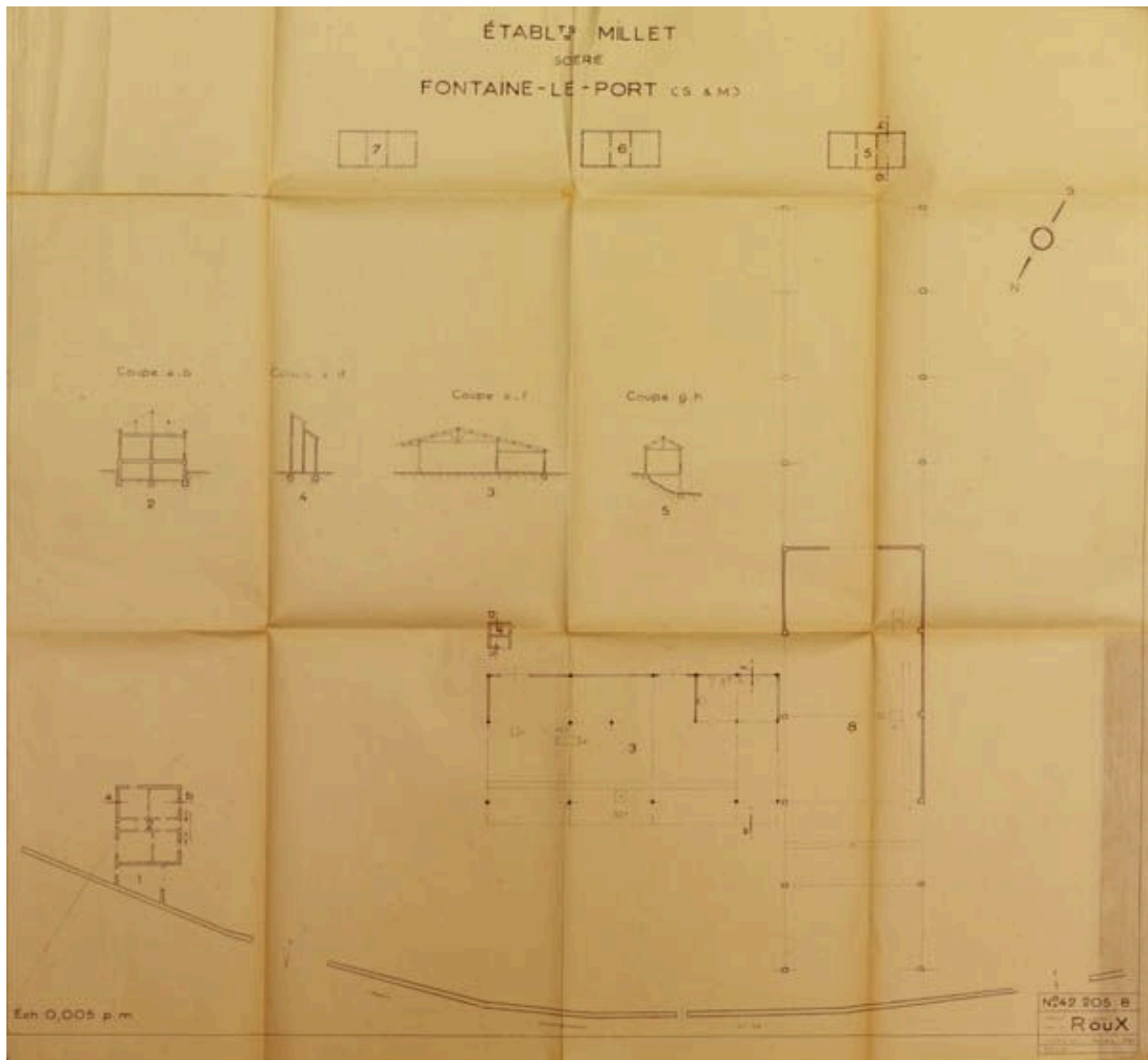
Plan-masse des établissements Millet (1947). (Collection particulière)
