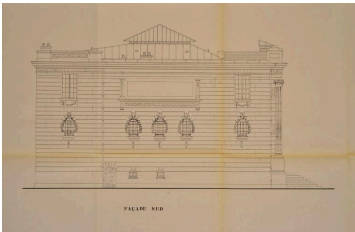
Relevé de la façade sud. Projet de restauration en 1981. Tirage. (AM Mantes-la-Jolie 53 W 123)
