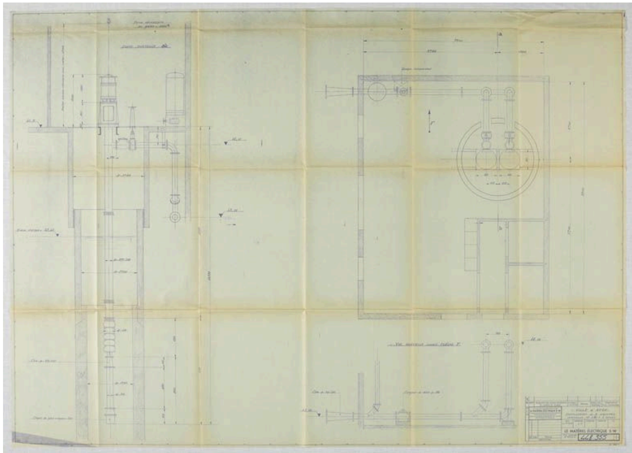
Plan et coupe des groupes électro-pompes installés à la station de pompage de Valvins par Le Matériel électrique S-W en 1954. (AD Seine-et-Marne, 3353W1169 )
