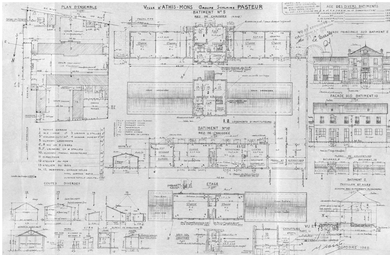
Plan d'ensemble, plans du rez-de-chaussée et du 1er étage des deux corps de bâtiment, élévations et coupes diverses ; octobre 1948.
