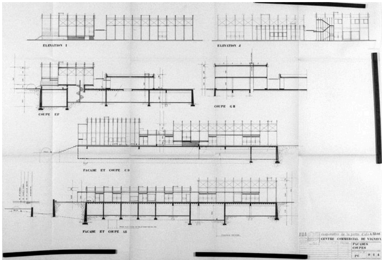
Façades, coupes. (AM Vigneux-sur-Seine, 80 W 22)
