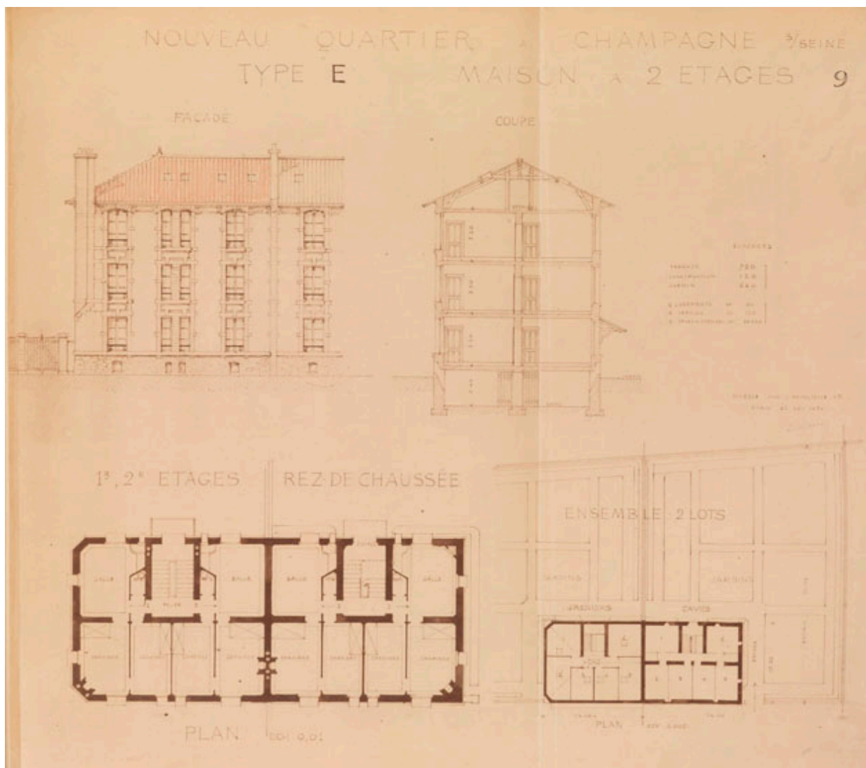
Edmond Delaire. Projet pour "le nouveau quartier" de Champagne-sur-Seine. Type E, maison à deux étages.
