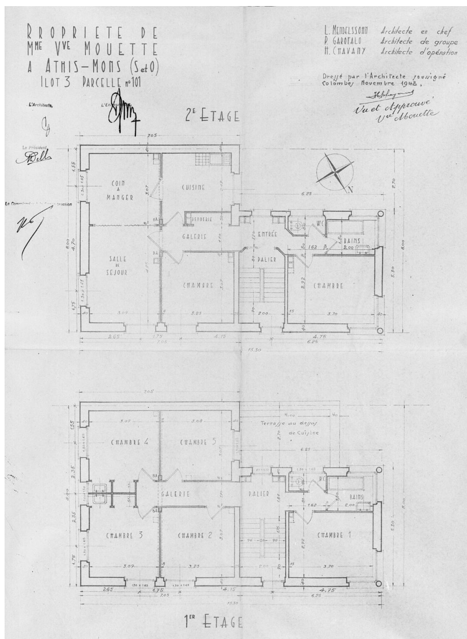
Plans des 1er et 2e étages de l'immeuble avec café en rez-de-chaussée reconstruit dans l'îlot 3 (parcelle 101) pour Mme Vve Mouette ; architecte en chef Léo Mendelssohn, P. Garofalo, architecte chef de groupe et H. Chavany, architecte d'opération, novembre 1948.
