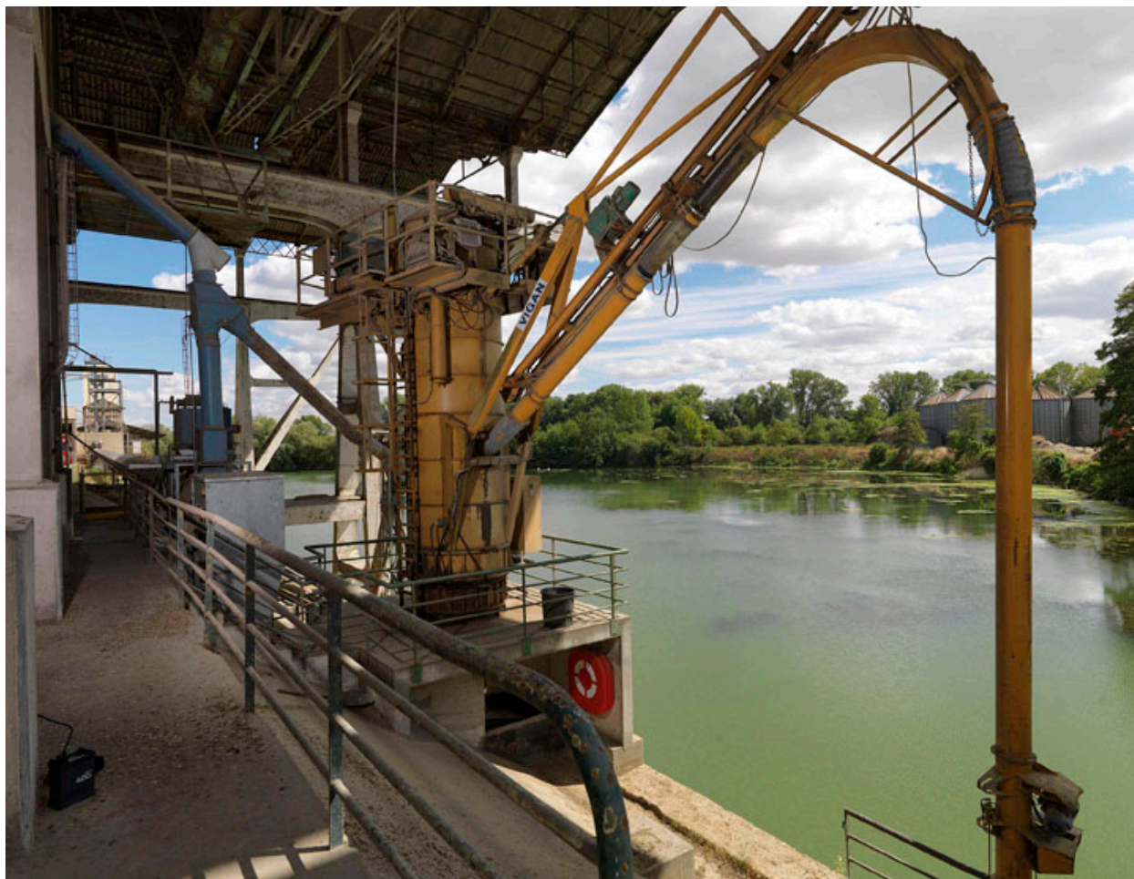
Silos de l'UNCAC de la Grande Paroisse, aujourd'hui Invivo. Silo 1. Aspirateur pneumatique a grain. au fond, la dars.
