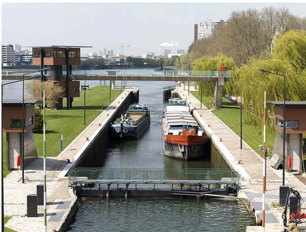
Alfortville, Vitry-sur-Seine. Barrage éclusé de Port-à-l'Anglais. Péniches dans l'écluse.
