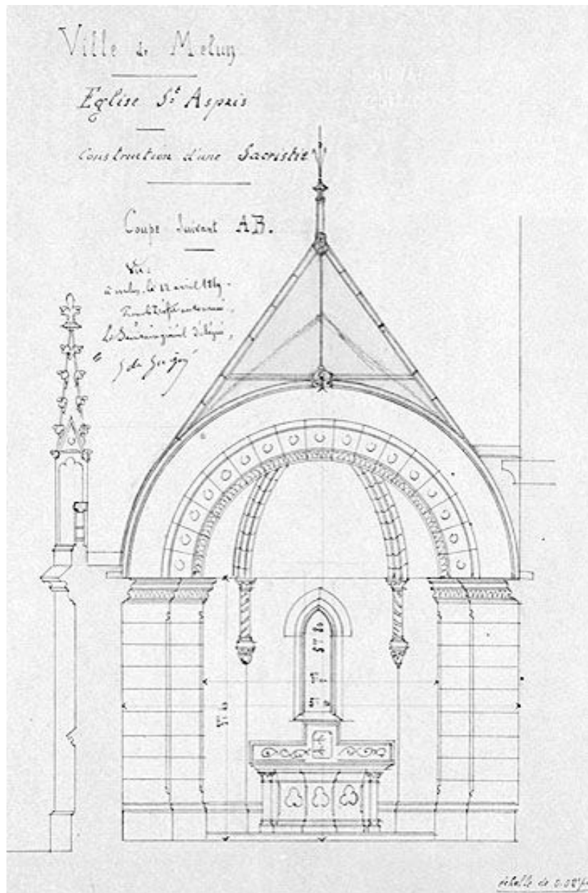
Ville de Melun. Eglise Saint-Aspais. Construction d'une sacristie. Coupe transversale. Echelle : 0.02 m.p.m. Calque aquarellé, 1869. (BM Melun. HH 25)
