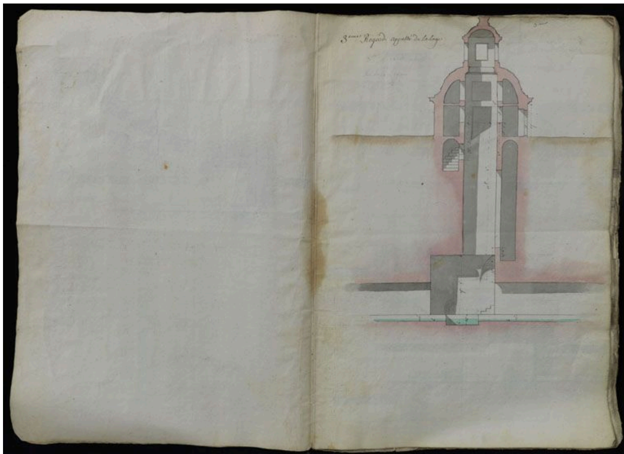
Fresnes. Coupe du regard III. Plans, 1765-1789. (Bibliothèque de l'Ecole de Nationale des Ponts et Chaussées, Ms.2567 -vol 2)
