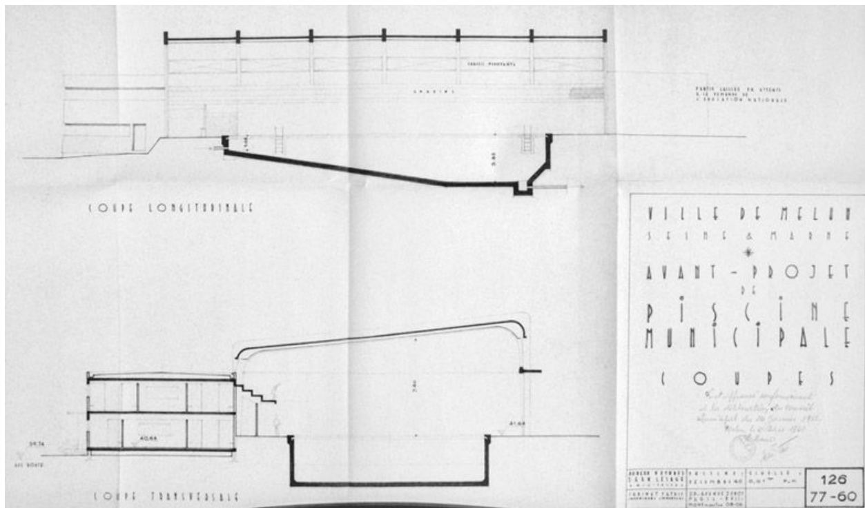
Coupes. Tirage d'architecte, décembre 1960. (AM Melun. 145 W 1)
