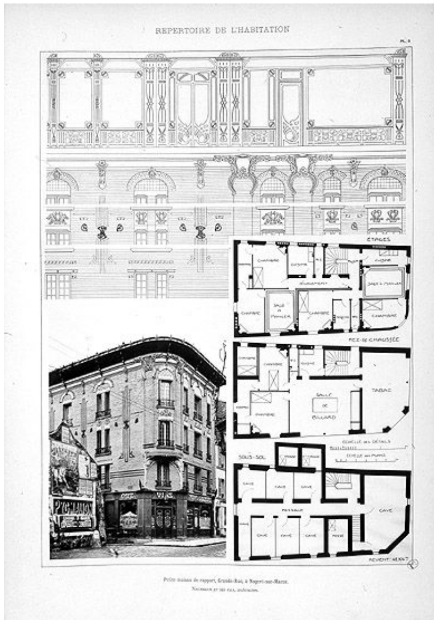
Plans, élévation et photographie d'une petit immeuble de rapport à Nogent-sur-Marne. Nachbaur, architecte. Tiré de : Répertoire de l'habitation / Th. Lambert, Paris : Ch. Massin, [191?]. (BHVP)
