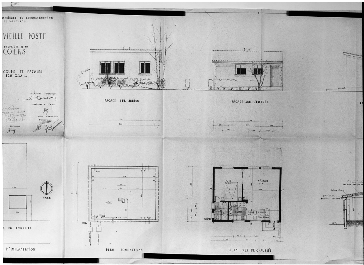
Plans et élévations du pavillon reconstruit pour M. Colas, allée des Fauvettes ; 21 décembre 1953.
