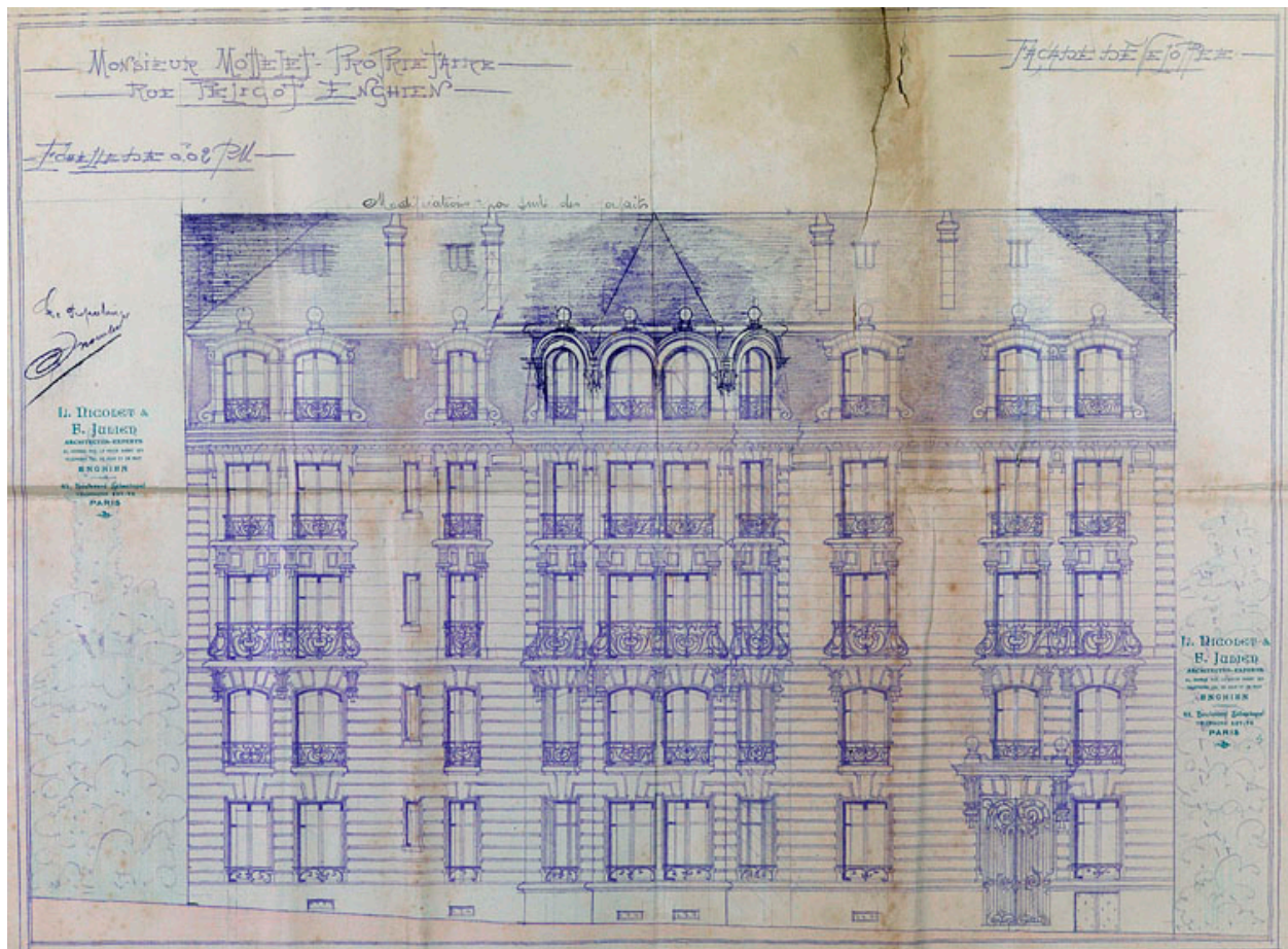
Élévation de la façade projetée de l'immeuble construit pour monsieur Mottelet vers 1910, à l'angle de la rue Pélégot et rue du Temple. (AM Enghien-les-Bains, Fonds des autorisations de permis de construire)
