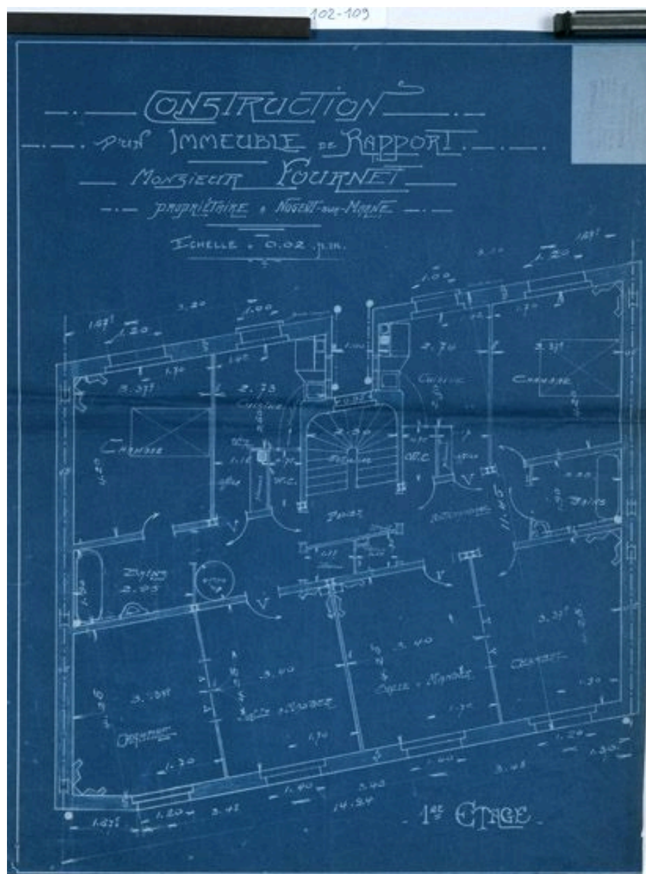
Plan de demande d'autorisation de construire d'un immeuble, Grande rue Charles de Gaulle. (AM Nogent-sur-Marne. 1 02 109)
