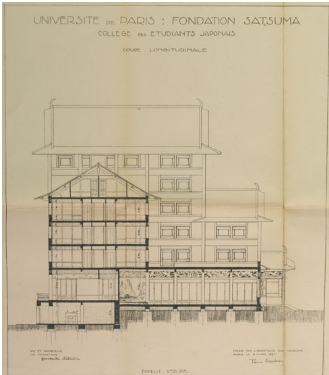
Coupe longitudinale par l'architecte Pierre Sardou, 5 avril 1927. Dessin. Archives nationales, 20090013/388.
