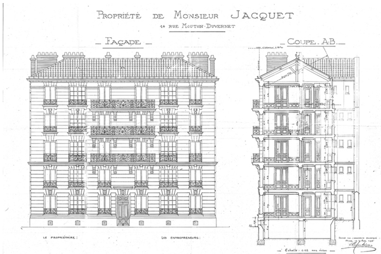
Facade et coupe, 14 rue Mouton Duvernet, propriété de M.Jacquet.- Plan, 1905. (Archives de Paris. VO11 2486).
