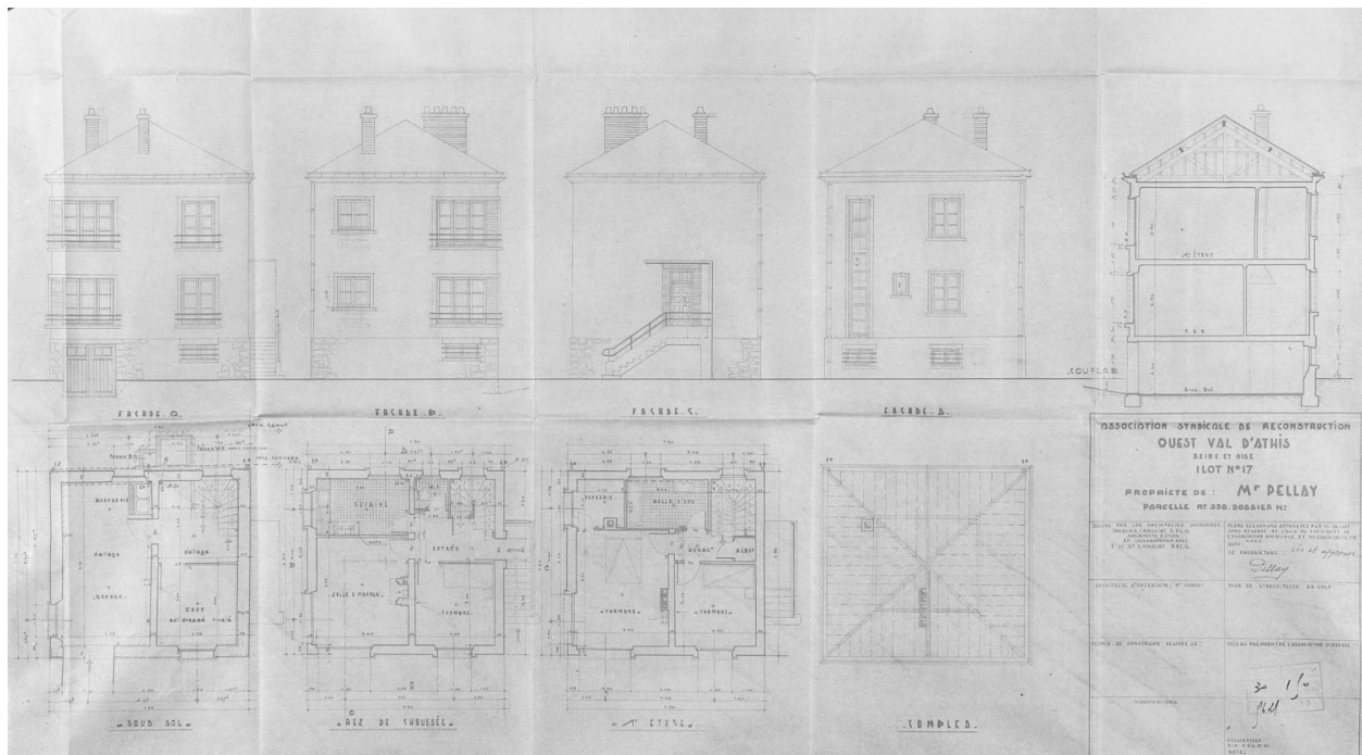
Elévations, coupes et plans de la maison reconstruite dans l'îlot 17 pour M. Pella, par J. et J.-P. Chauliat, s. d.
