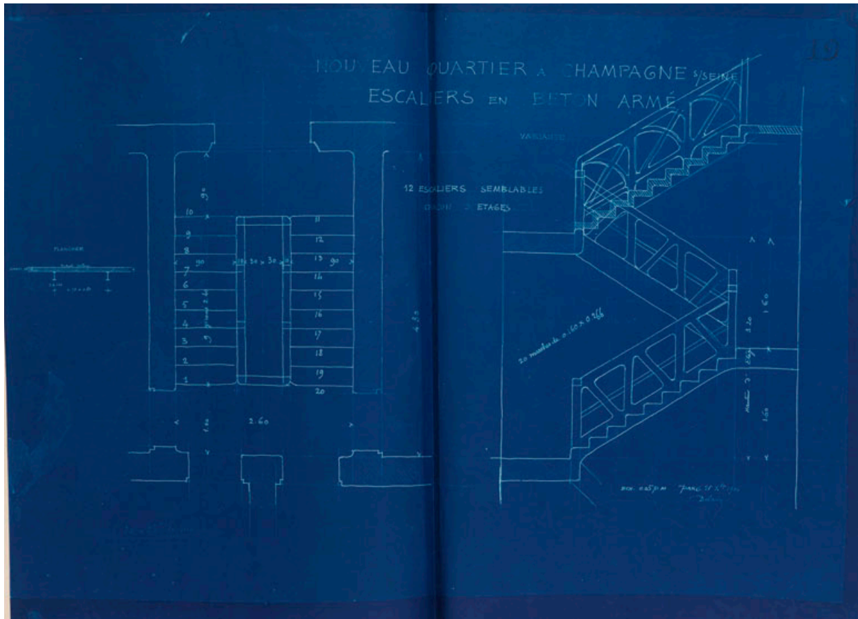
Plan. Edmond Delaire. Projet pour "le nouveau quartier" de Champagne-sur-Seine. Escalier en béton armé.
