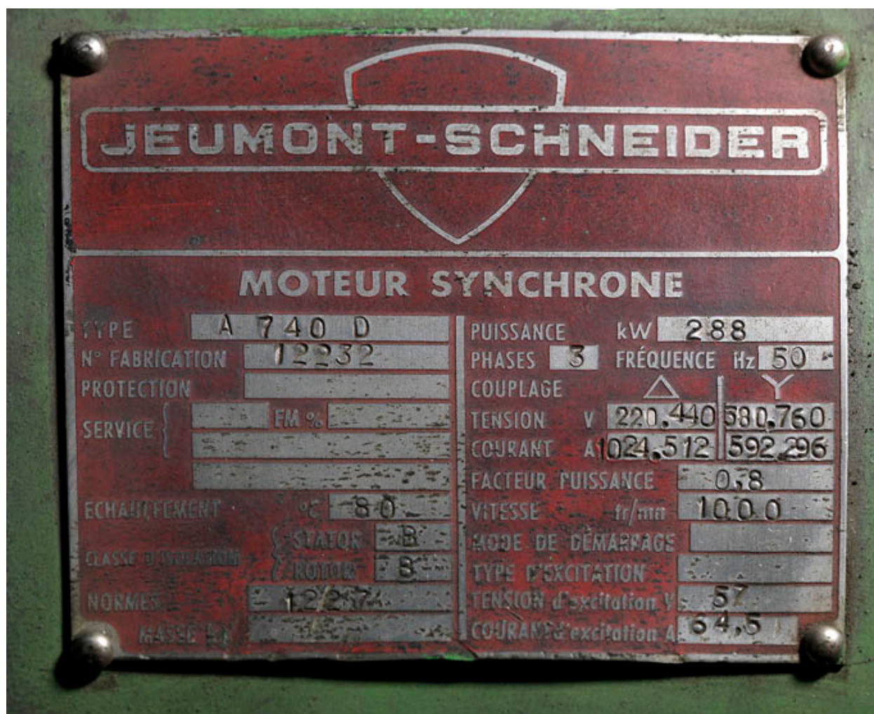
Plateforme d'essais. Entreprise Jeumont-Electric. Plaque d'identification d'un moteur synchrone Jeumont-Schneider.
