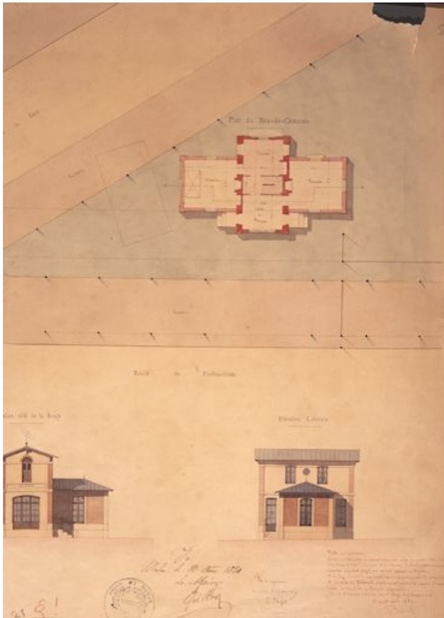
Projet de construction d'un bâtiment d'octroi à la barrière de Fontainebleau : plan et élévations. Papier aquarellé, 08 août 1850. (AM Melun. 1 Fi 548 (partie droite du document))
