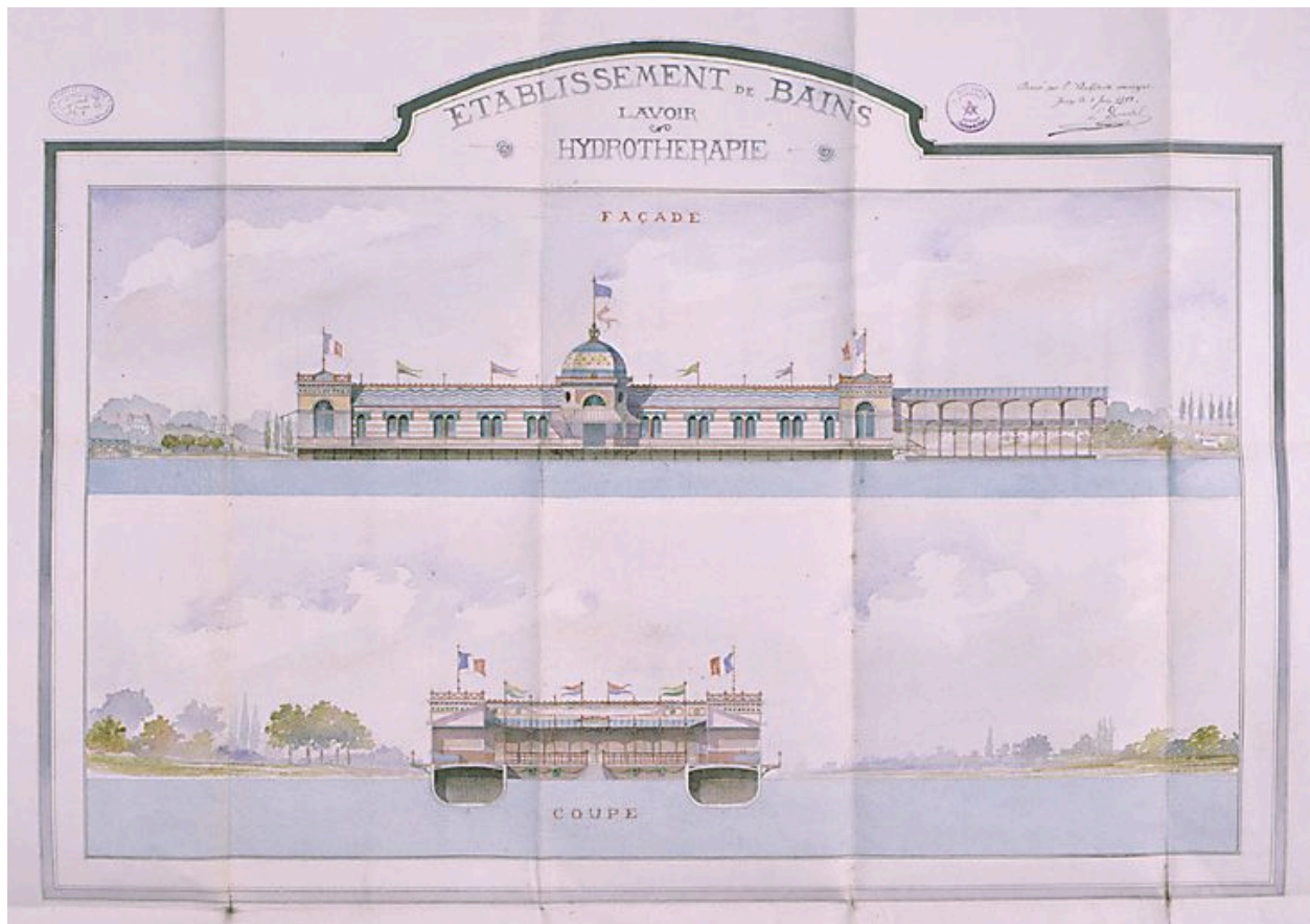
Projet d'installation en Seine sur la rive de Draveil d'un établissement de bains-douches, d'un lavoir et d'un bassin de natation : élévation longitudinale et coupe transversale, planche aquarellée, datée 1893 et signée L. Ducastel. (AD Essonne, 3 S 26)
