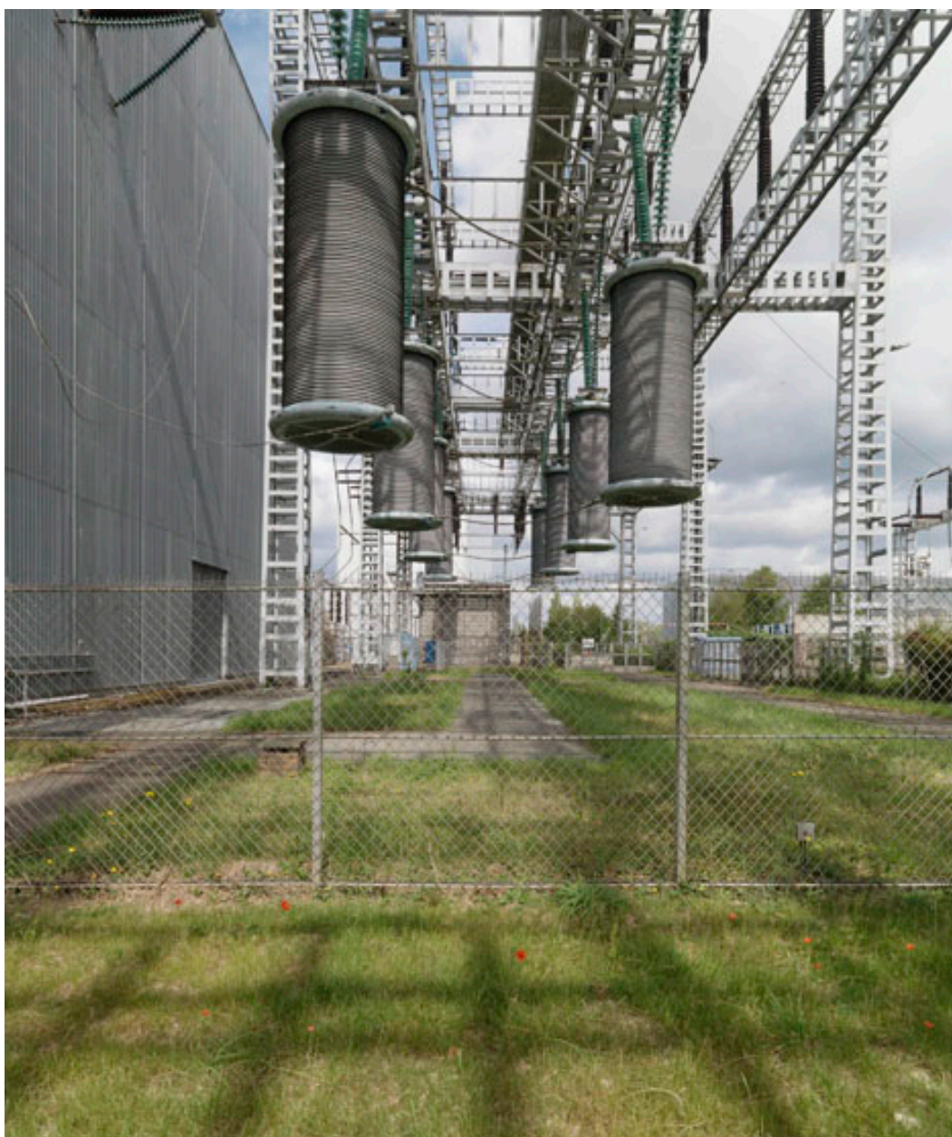
Charpente électrique extérieure. Détail. A gauche le Hall d'essais synthétiques.
