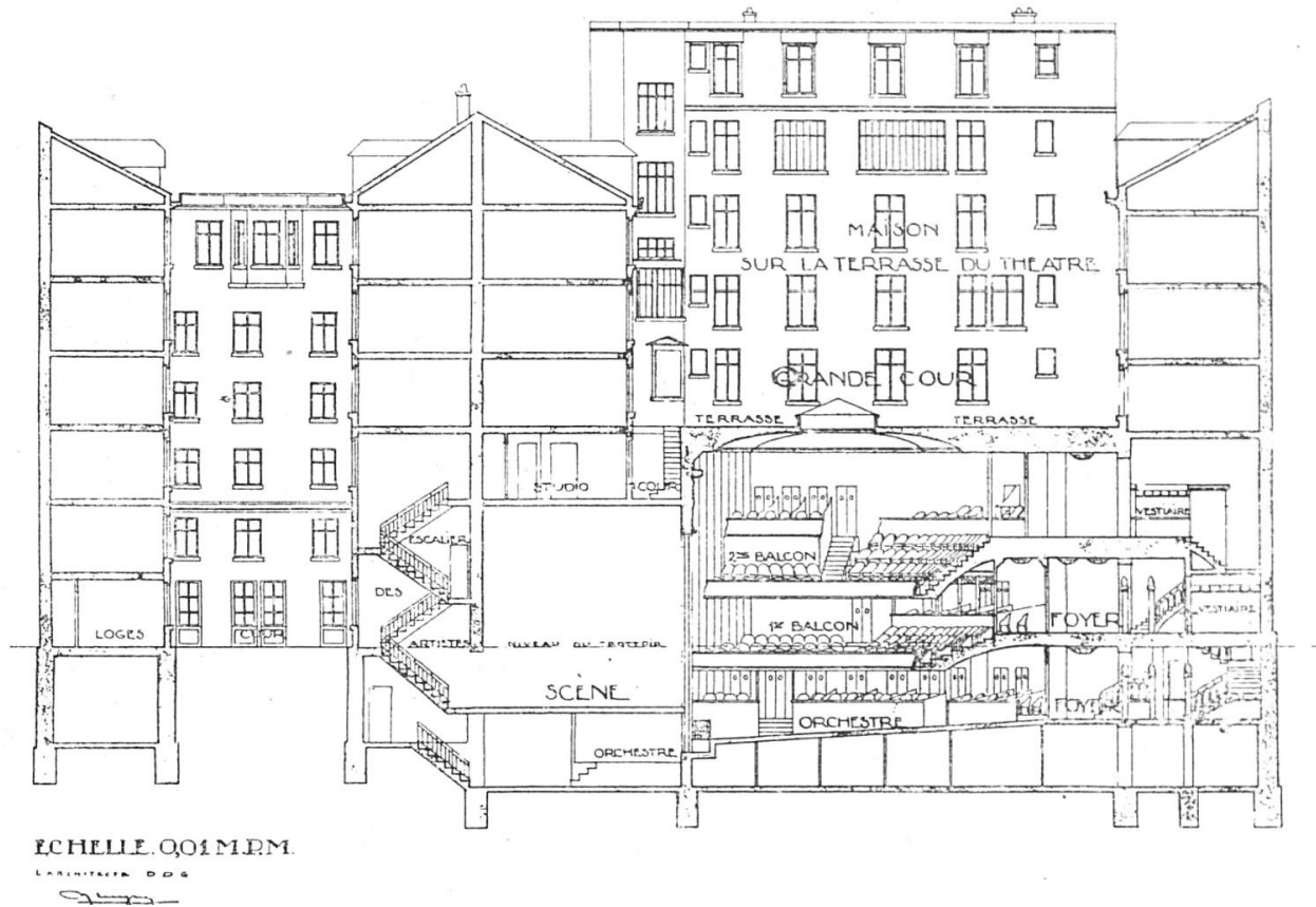
Coupe longitudinale (L'Architecture, 1927)
