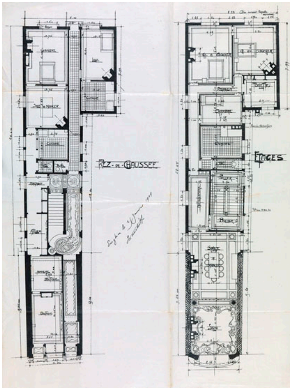
Plans du rez-de-chaussée et des étages (1904) (AM Enghien-les-Bains)
