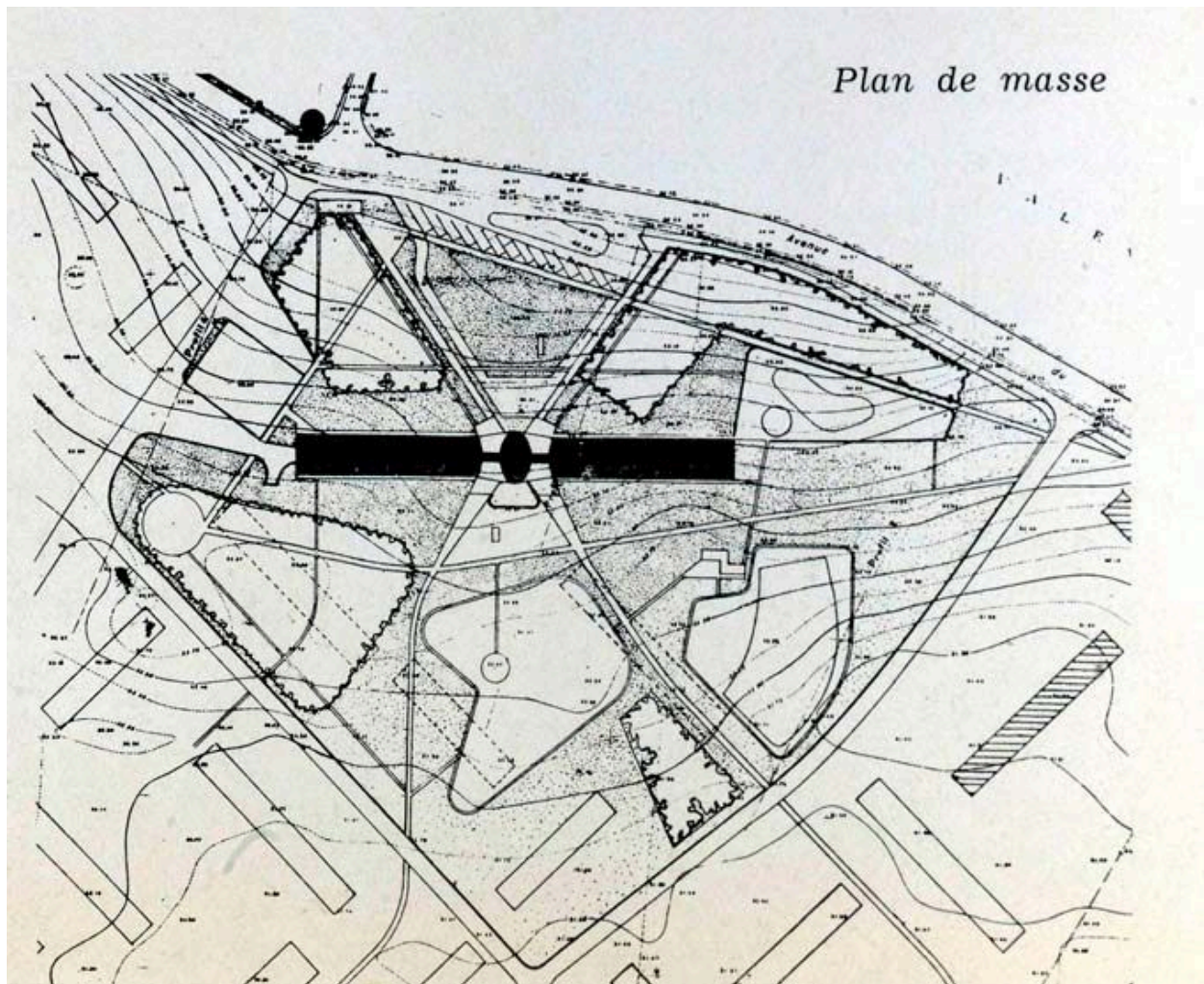
Villeneuve-Saint-Georges, cité dite cité Gabriel Péri, avenue Division Leclerc, Cité des Tours. Plan masse de l'un des projets. Tiré de : Villeneuve-Saint-Georges, cité Gabriel Péri. Présentation des différents projets. In Architecture française, n° 103-104, 1950.
