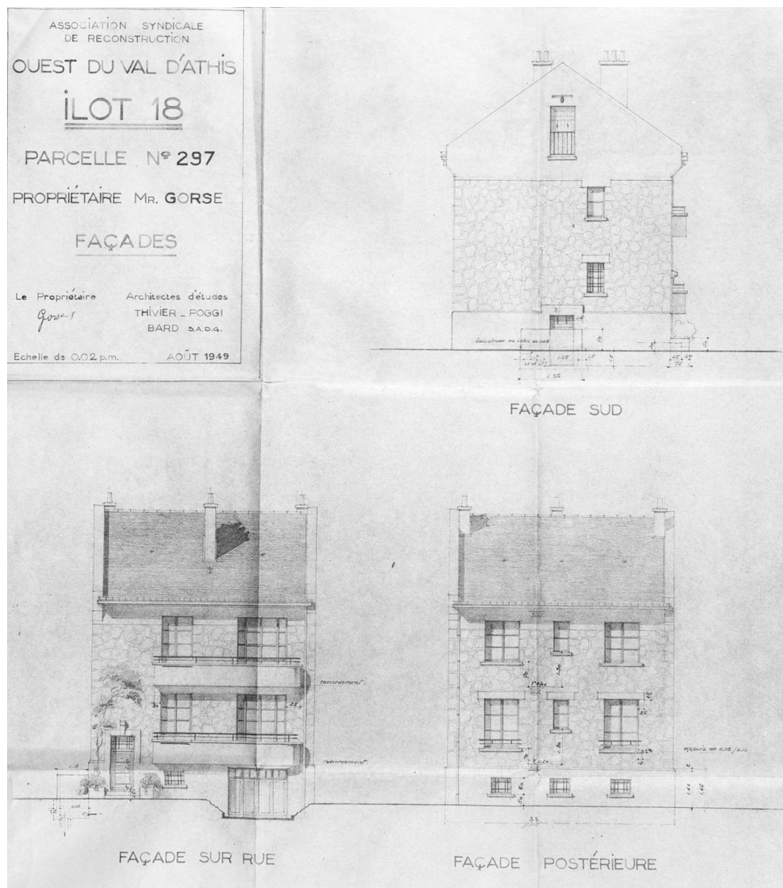
Façades de la maison reconstruite sur la parcelle 297 de l'îlot 18 pour M. Gorse (14, rue Bertrand-Maupomé), par Thivier et Poggi et Bard, architectes d'études, août 1949.
