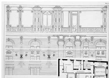
Détail des élévations d'un petit immeuble de rapport à Nogent-sur-Marne. Nachbaur, architecte. Tiré de : Répertoire de l'habitation / Th. Lambert, Paris : Ch. Massin, [191?]. (BHVP) IVR11_20059400313XA
