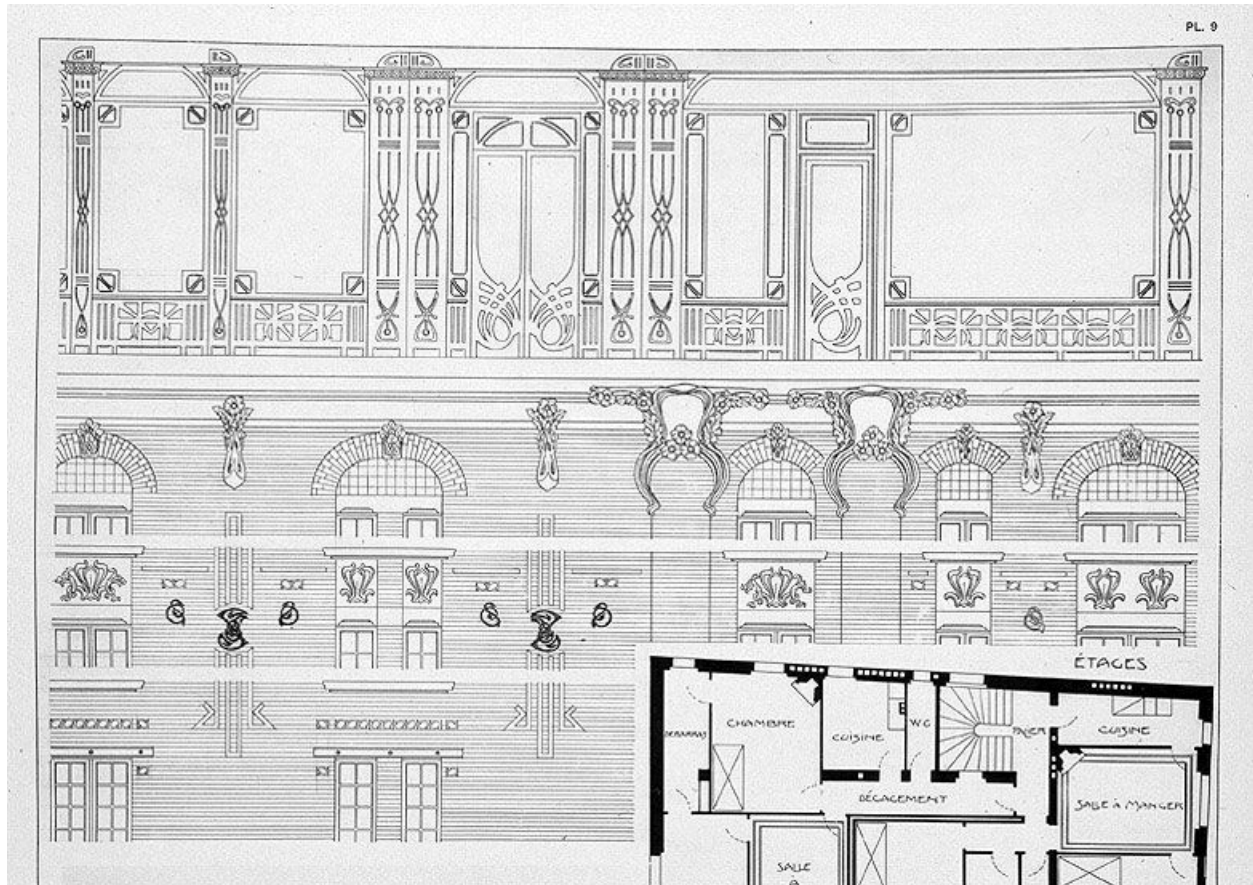
Détail des élévations d'un petit immeuble de rapport à Nogent-sur-Marne. Nachbaur, architecte. Tiré de : Répertoire de l'habitation / Th. Lambert, Paris : Ch. Massin, [191?]. (BHVP)
