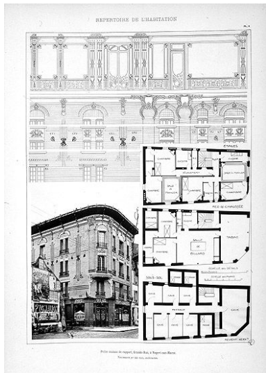
Plans, élévation et photographie d'une petit immeuble de rapport à Nogent-sur-Marne. Nachbaur, architecte. Tiré de : Répertoire de l'habitation / Th. Lambert, Paris : Ch. Massin, [191?]. (BHVP) IVR11_20059400309XA
