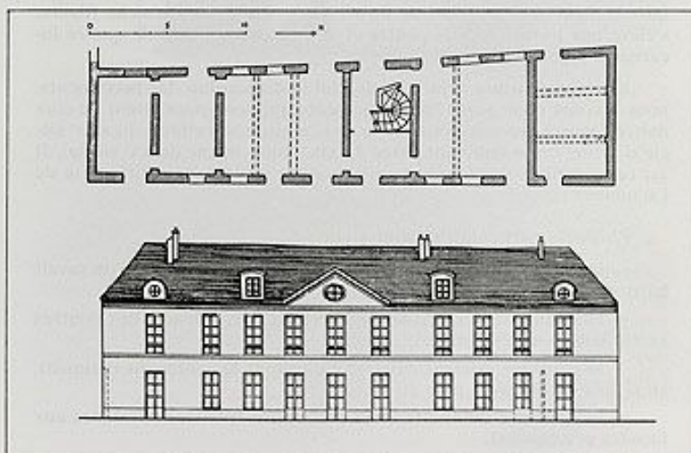
Fig. 5. — Plan du rez-de-chaussée et façade Est : essai de restitution (J.-L. GUENOUN, 1985)
