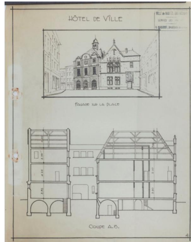
Elevation et coupe de l'hôtel de ville et auditoire vers 1940. AM. Mantes-la-Jolie, 1 M 1. Phot. Laurent Kruszyk IVR11_20177800482NUC4A
