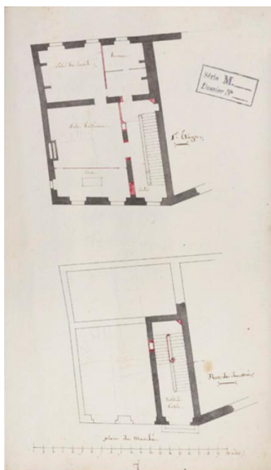
Plan de l'hôtel de ville au début du XIXe siècle. Le rez-de-chaussée. AM Mantes-la-Jolie, 1 M 3. Phot. Laurent Kruszyk IVR11_20177800520NUC4A
