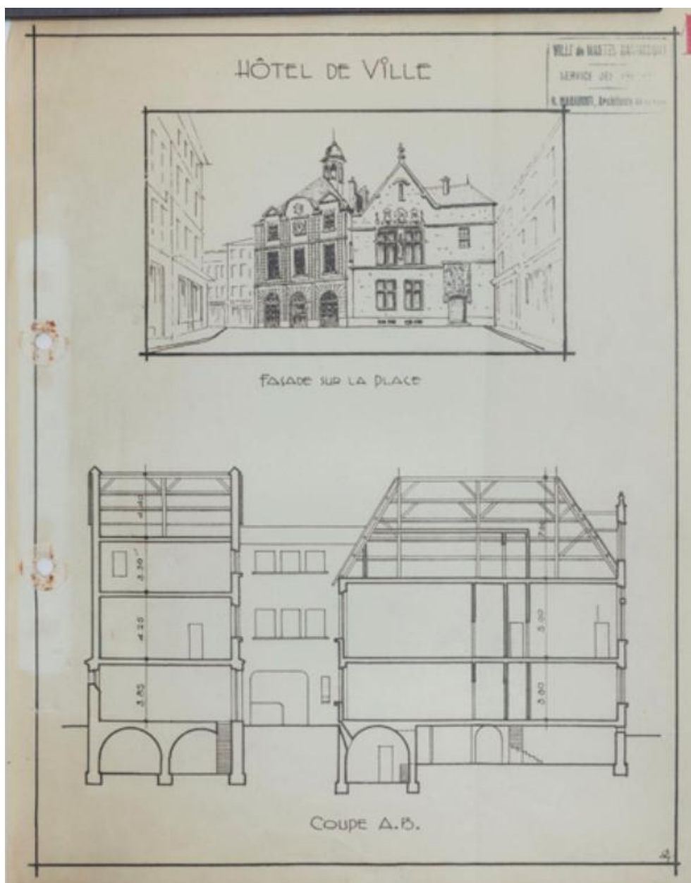
Elevation et coupe de l'hôtel de ville et auditorio vers 1940. AM. Mantes-la-Jolie, 1 M 1.
