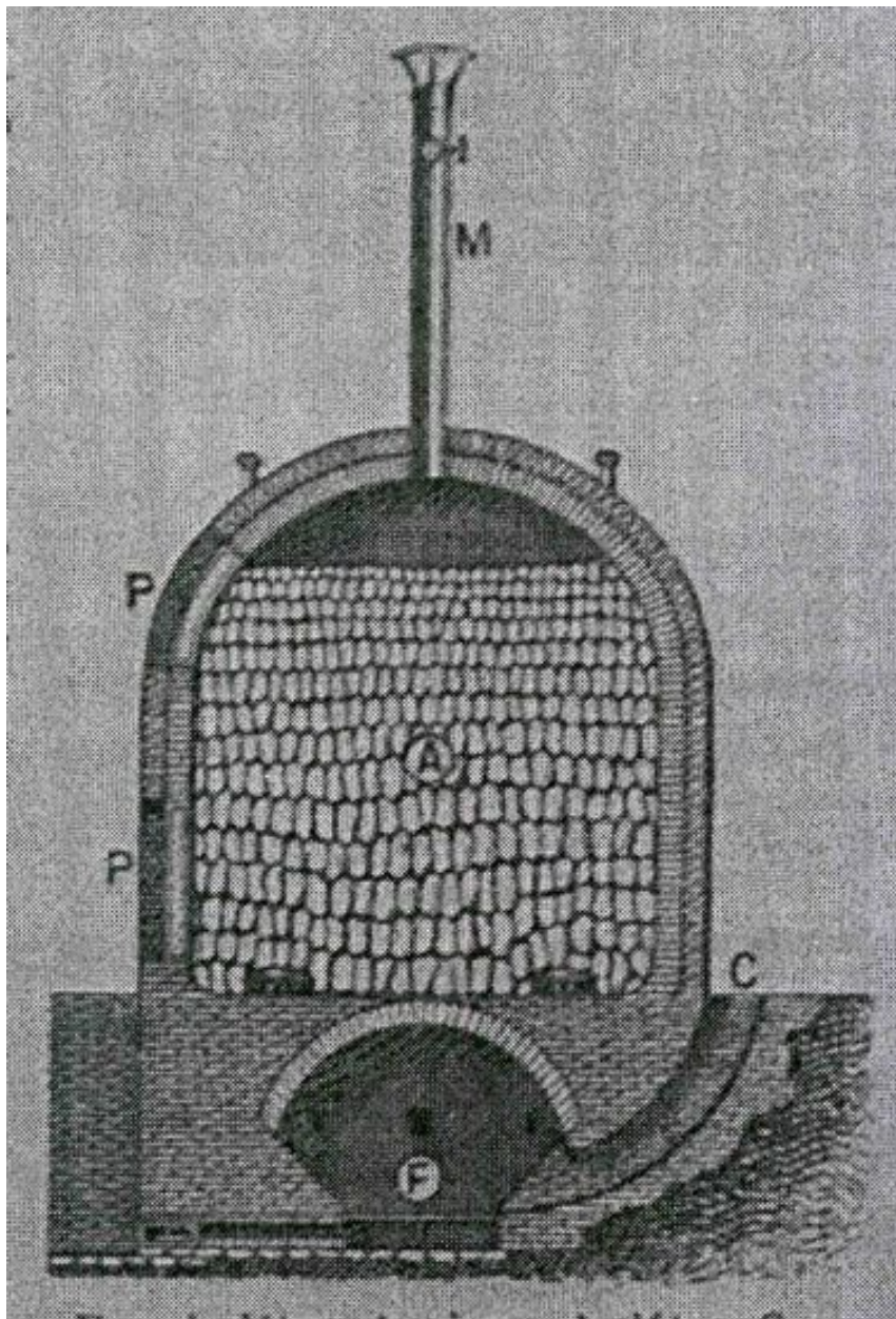
Dessin représentant, en coupe, un four vertical en usage au tournant du 19e et du 20e siècle. Tiré de : "Dictionnaire encyclopédique Larousse, 1909.
