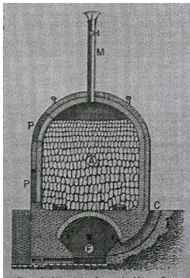
Dessin représentant, en coupe, un four vertical en usage au tournant du 19e et du 20e siècle. Tiré de : "Dictionnaire encyclopédique Larousse, 1909. IVR11_20097701563XA
