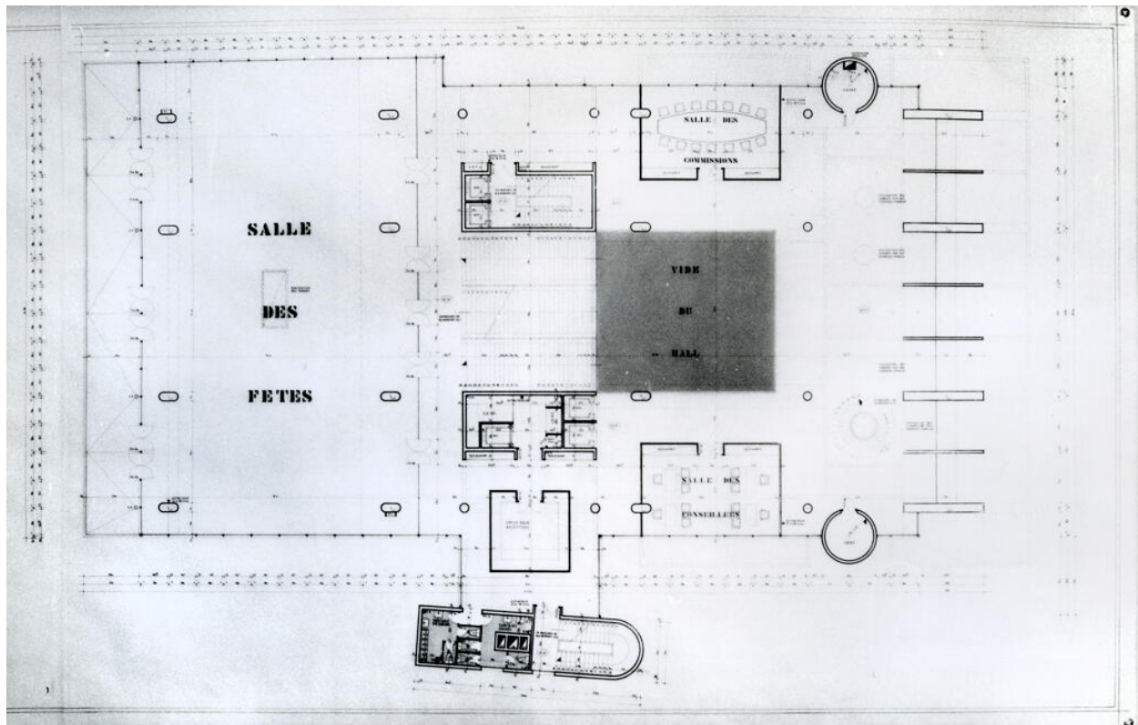
Plan du premier étage, projet, dessin [s. d.]. Tirage photographique noir et blanc (reproduction), 18 x 24 cm, s. d. [vers 1976], (coll. Gilbert Picquenard).
