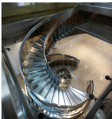
Vue de l'escalier en vis desservant les bureaux du deuxième étage. Limon, rampes et marches en acier inoxydable, garde- corps en verre fumé. Conçu par G. Picquenard, construit par l'entreprise Voisin (fabrication en atelier, puis remonté sur place). Phot. Asseline Stéphane IVR11_20249400422NUC4A
