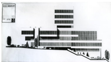
Élévation de de la façade sud, projet, dessin [s. d.]. Tirage photographique noir et blanc (reproduction), 18 x 24 cm, s. d. [vers 1976], Louis Martin, Saint-Maur, (coll. Gilbert Picquenard). IVR11_20249400474NUC4A
