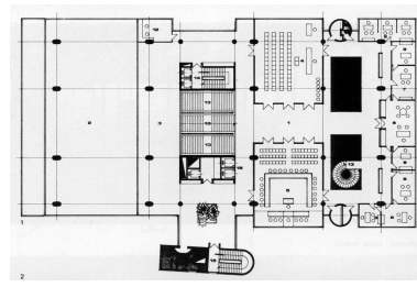
Plan du deuxième étage, publié dans "Centre administratif - Hôtel de ville à Joinville-le-Pont, Robert et Gilbert Picquenard architectes", dans "Recherche & Architecture", n° 30, 1977, p. 44 (coll. Gilbert Picquenard). IVR11_20249400488NUC4A
