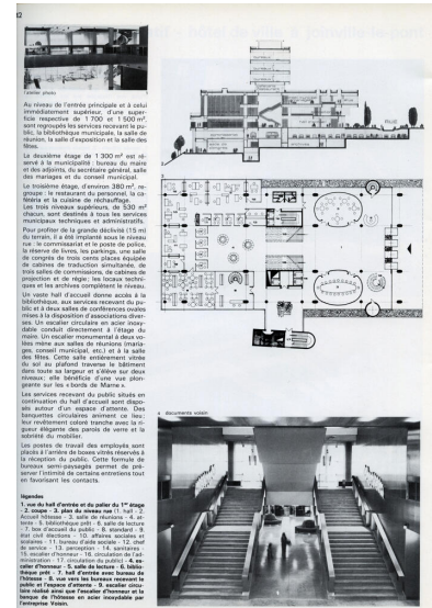
"Centre administratif - Hôtel de ville à Joinville-le-Pont, Robert et Gilbert Picquenard architectes", dans "Recherche & Architecture", n° 30, 1977, p. 42 (coll. Gilbert Picquenard). IVR11_20249400482NUC4A
