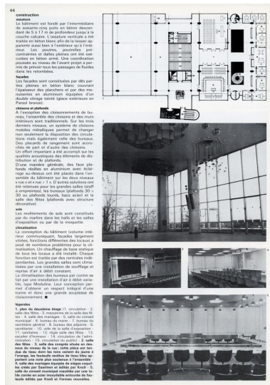
"Centre administratif - Hôtel de ville à Joinville-le-Pont, Robert et Gilbert Picquenard architectes", dans "Recherche & Architecture", n° 30, 1977, p. 44 (coll. Gilbert Picquenard). IVR11_20249400484NUC4A
