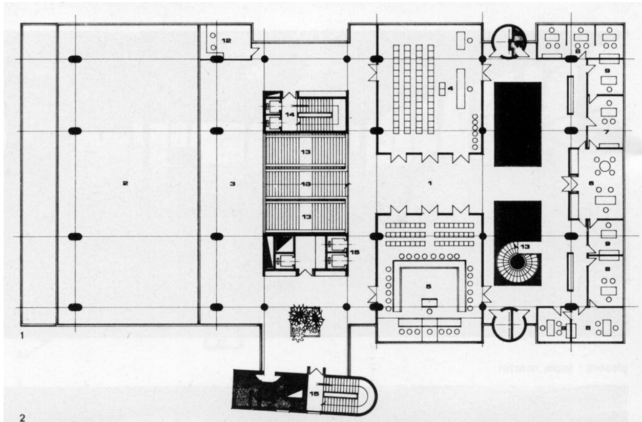
Plan du deuxième étage, publié dans "Centre administratif - Hôtel de ville à Joinville-le-Pont, Robert et Gilbert Picquenard architectes", dans "Recherche & Architecture", n° 30, 1977, p. 44 (coll. Gilbert Picquenard).
