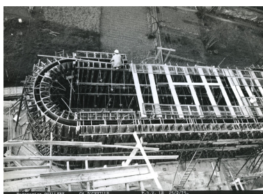
Mise en place du coffrage de l'escalier hors-œuvre. Tirage photographique noir et blanc, 18 x 24 cm, 25 février 1975, album de photographies de chantier réalisé par Gérard Guillaud - L'Image Contemporaine, pour l'entreprise Quillery (coll. Gilbert Picquenard).
