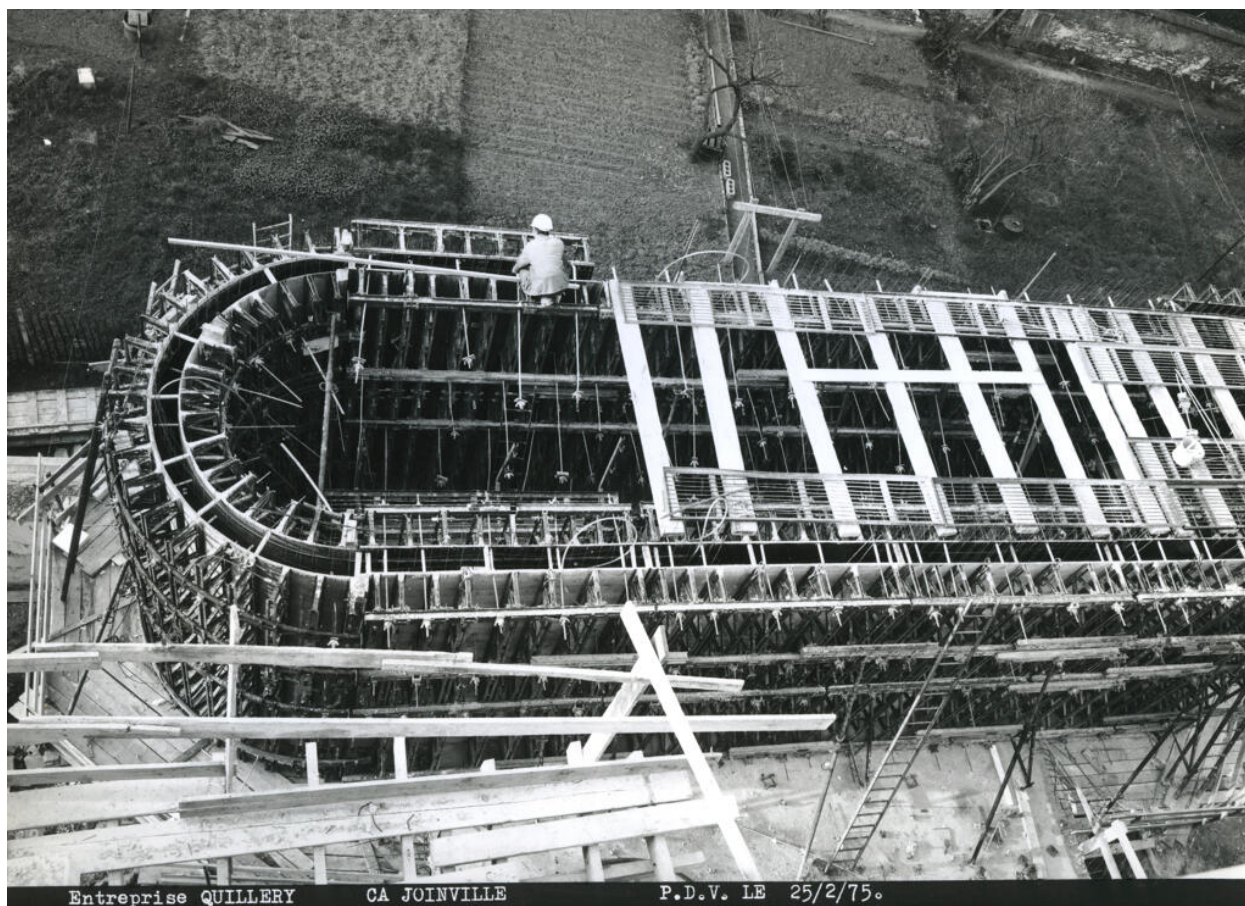
Mise en place du coffrage de l'escalier hors-œuvre. Tirage photographique noir et blanc, 18 x 24 cm, 25 février 1975, album de photographies de chantier réalisé par Gérard Guillet - L'Image Contemporaine, pour l'entreprise Quillery (coll. Gilbert Picquenard).
