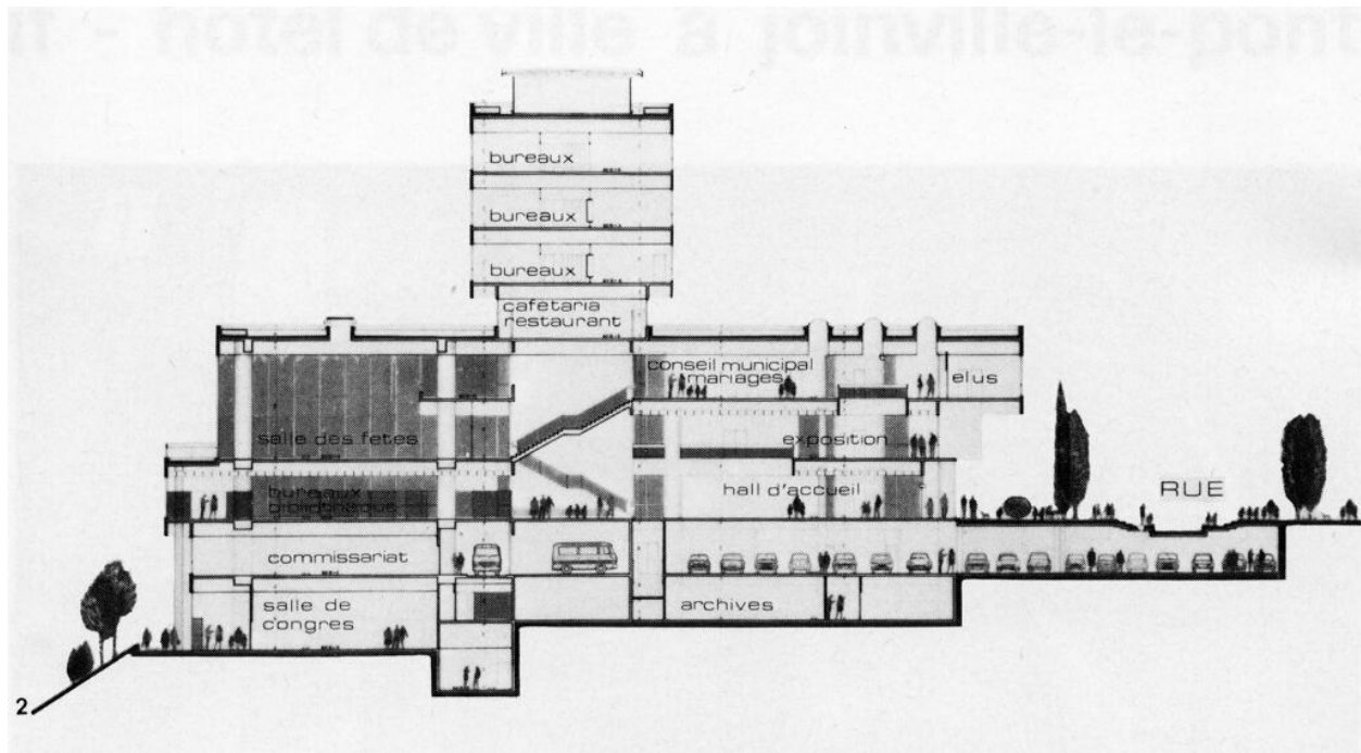
Coupe transversale, publiée dans "Centre administratif - Hôtel de ville à Joinville-le-Pont, Robert et Gilbert Picquenard architectes", dans "Recherche & Architecture", n° 30, 1977, p. 42 (coll. Gilbert Picquenard).
