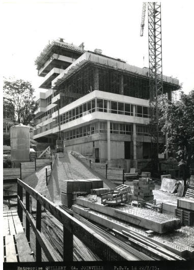
Vue de la façade nord en chantier. Tirage photographique noir et blanc, 18 x 24 cm, 22 juillet 1975, album de photographies de chantier réalisé par Gérard Guillet - L'Image Contemporaine, pour l'entreprise Quillery (coll. Gilbert Picquenard). IVR11_20249400458NUC4A
