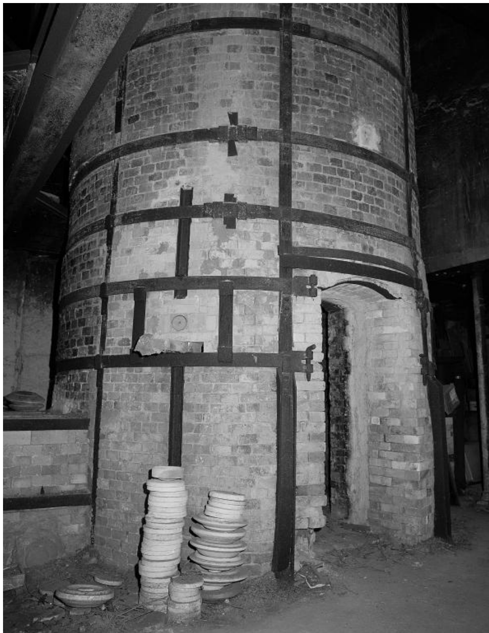
Embase et porte de l'un des fours. Photographie. (AD Seine-Saint-Denis. A NB 94)
