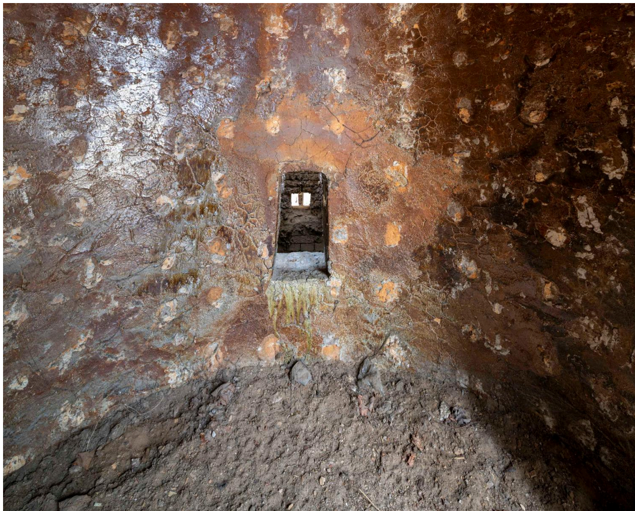
Intérieur du four rond à globe et à flamme renversée.
