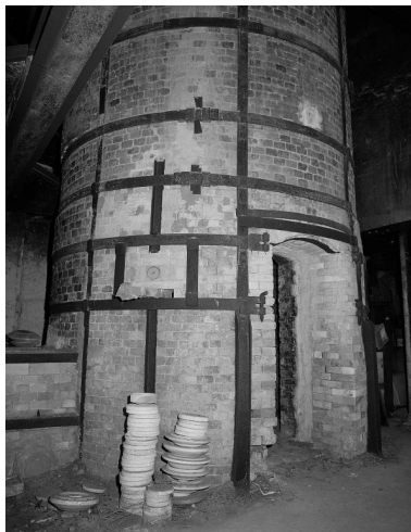
Embase et porte de l'un des fours. Photographie. (AD Seine-Saint-Denis. A NB 94) IVR11_20029300129NUC
