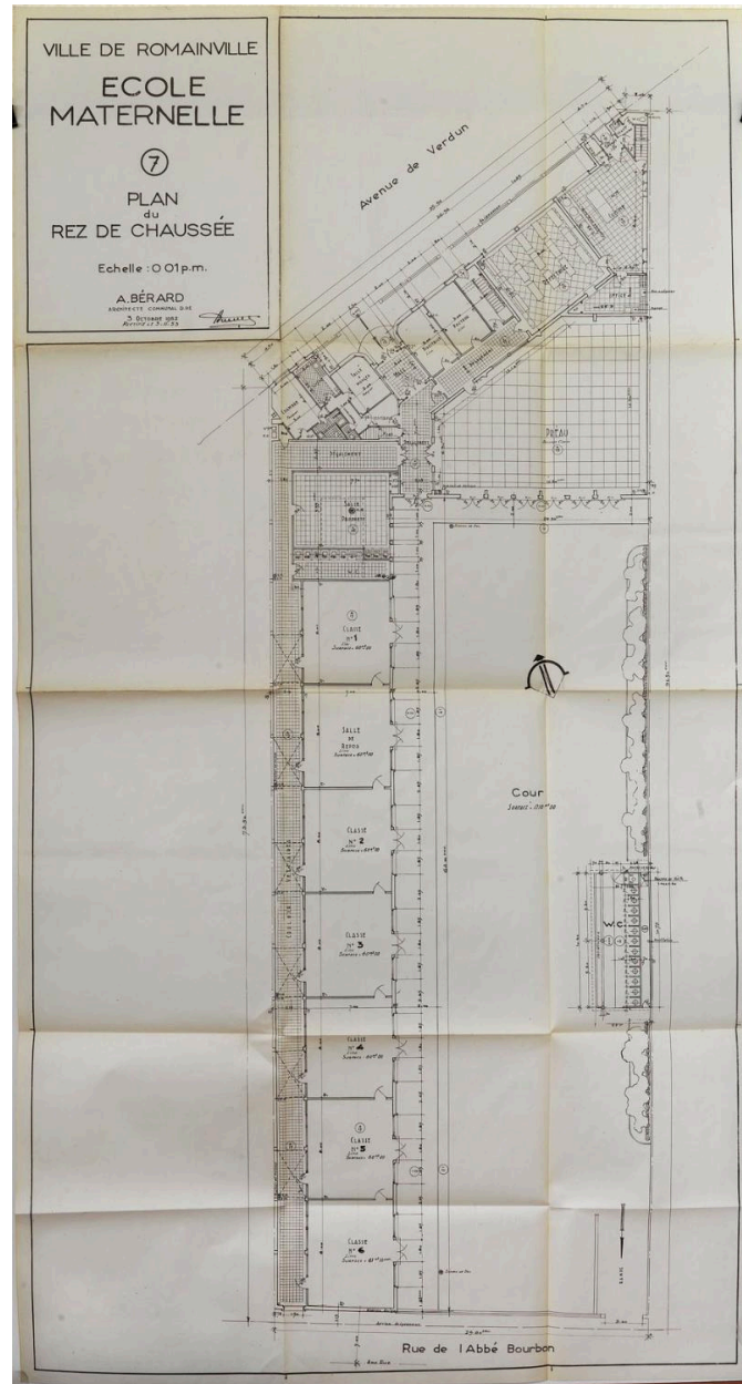
Plan du rez-de-chaussée. (AM Romainville)
