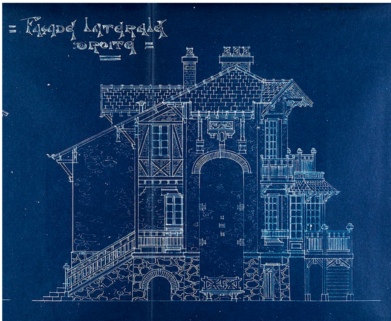
Détail de l'élévation de la façade latérale droite, 1907. (Institut français d'architecture, Fonds Hennebique Béton armé, BAH 3-1907-2467 )
