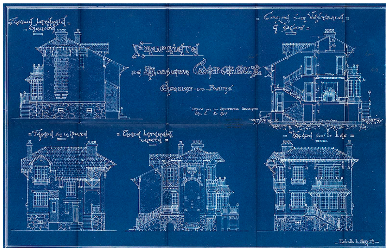
Elévations des quatre façades de l'édifice, 1907. (Institut français d'architecture, Fonds Hennebique Béton armé, BAH 3-1907-2467 )
