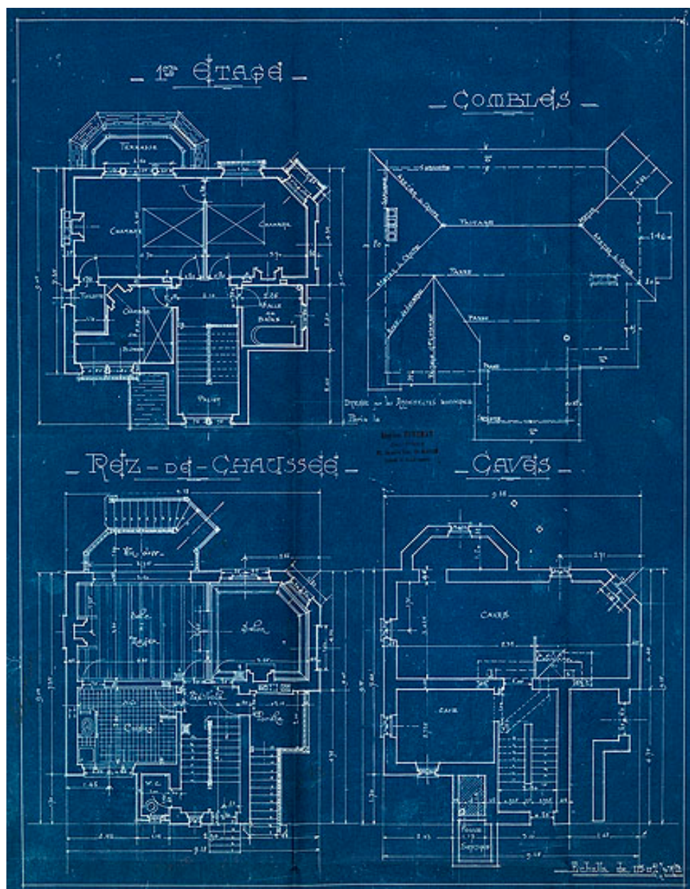
Plans du rez-de-chaussée, premier étage, combles et caves. 1907. (Institut français d'architecture, Fonds Hennebique Béton armé, BAH 3-1907-2467 )
