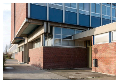
Lycée Rostand : le soubassement affiche la structure en béton, tandis que la façade écran la masque. Phot. Laurent Kruszyk IVR11_20177800313NUC4A
