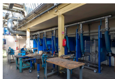
Lycée Rostand : l'atelier de la section Réalisations industrielles en Chaudronnerie et Soudures (RICS). Système d'aspiration pour les scories.
