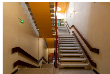
Lycée Rostand : on voit la large crémaillère qui soutient les marches et la forme incurvée de ces dernières, caractéristique des années 60. Phot. Laurent Kruszyk IVR11_20177800332NUC4A
