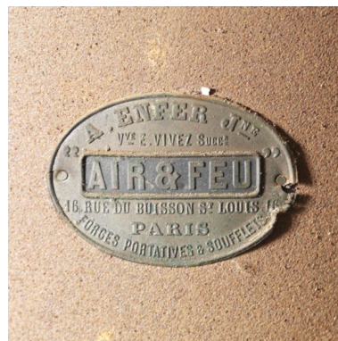
Soufflet à cylindres, détail de la plaque du fabricant. Phot. Chloé Bazaud IVR11_20097700067NUC4A
