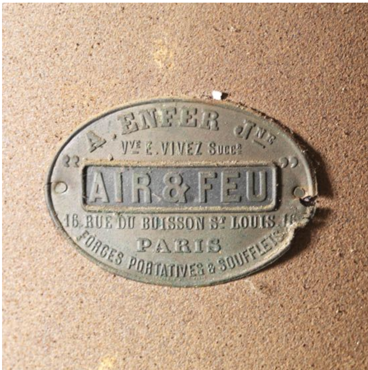
Soufflet à cylindres, détail de la plaque du fabricant.
