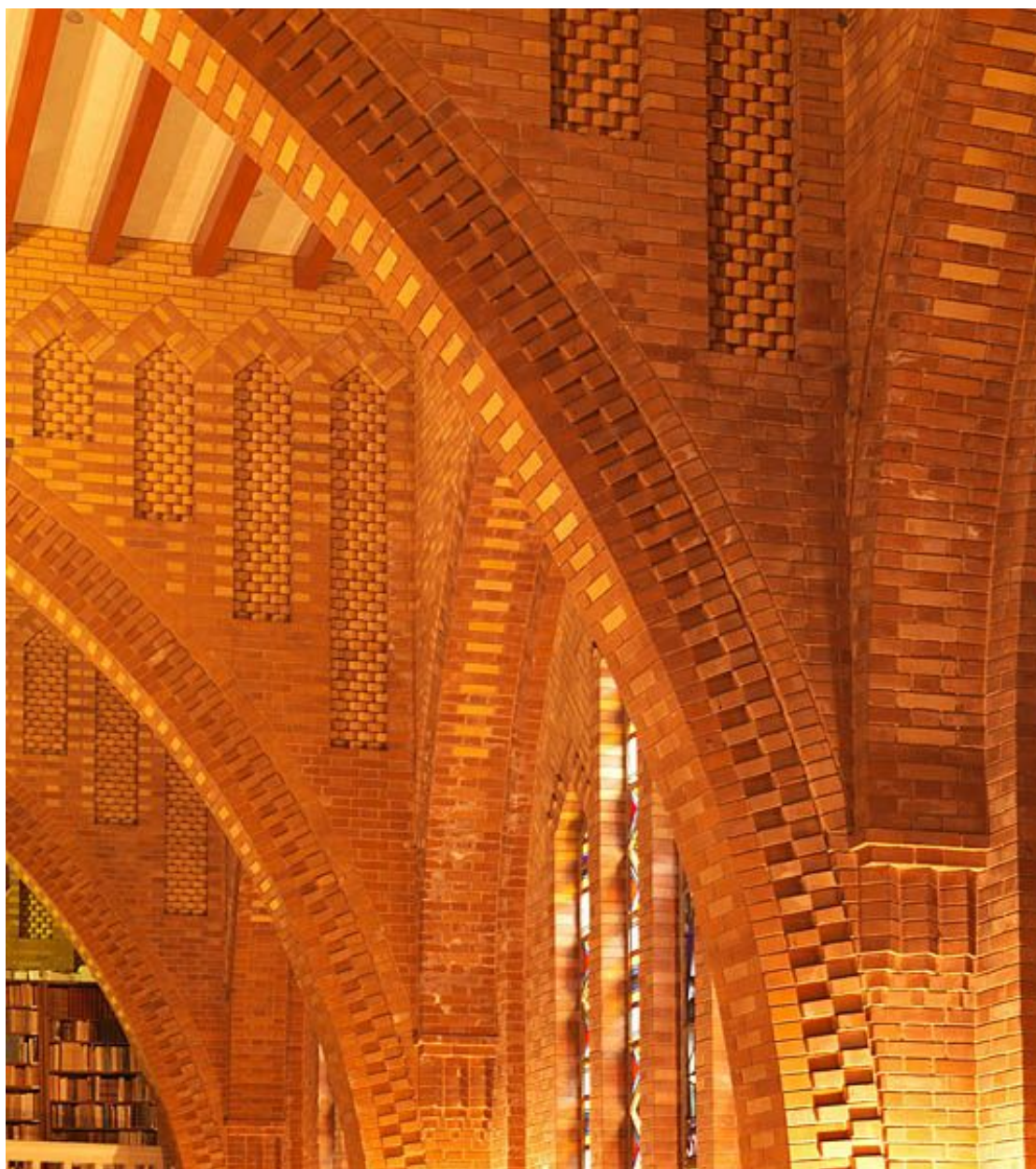
Chapelle de l'abbaye notre-Dame de Chaage. Détails de la mise en oeuvre du décor de brique.
