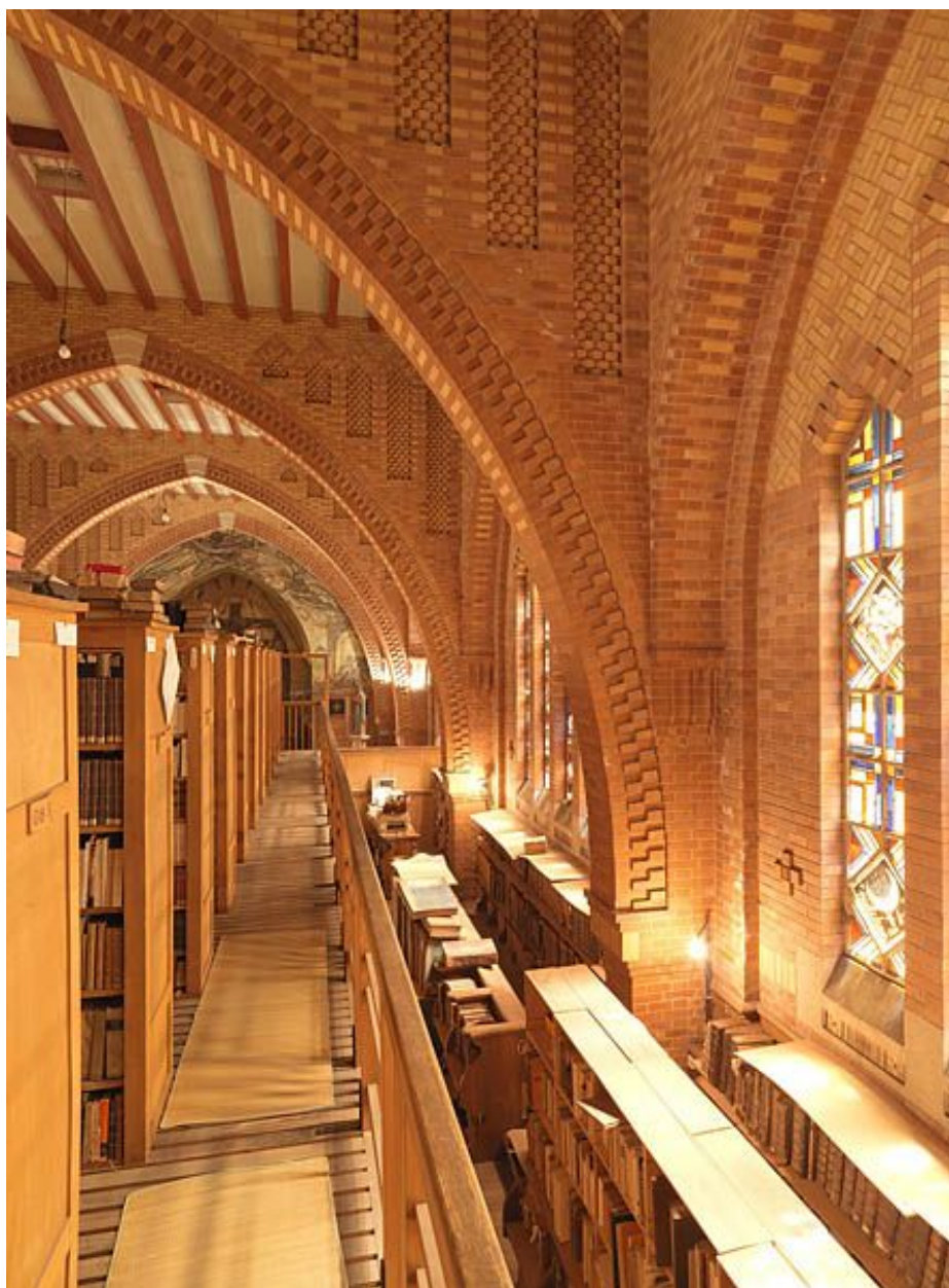
Chapelle de l'abbaye notre-Dame de Chaage. Détails de la mise en oeuvre des briques polychromes.
