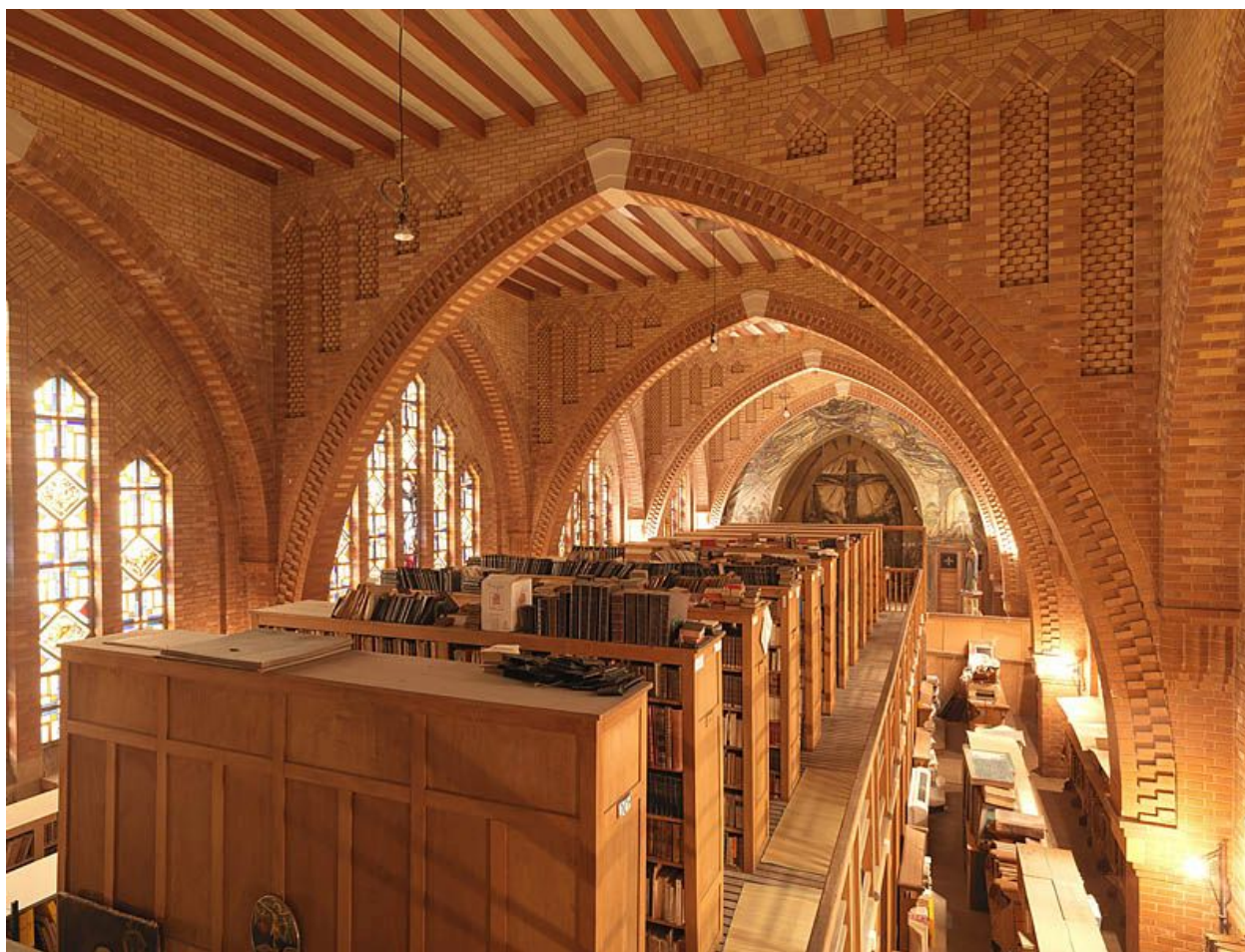
Chapelle de l'abbaye notre-Dame de Chaage. Vue perspective vers le chœur.
