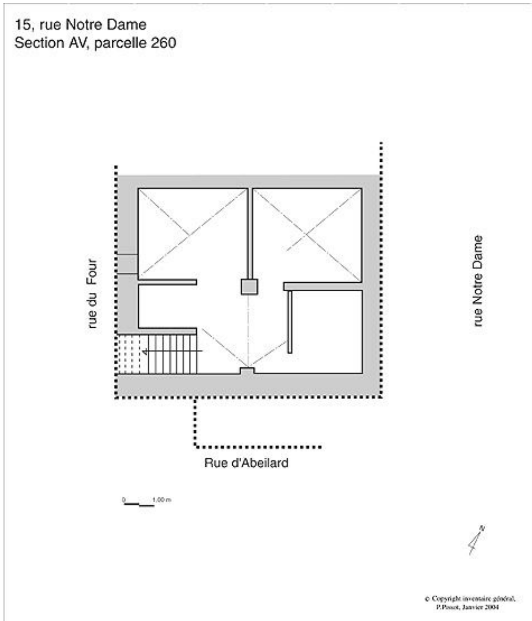
Plan schématique de la cave.
