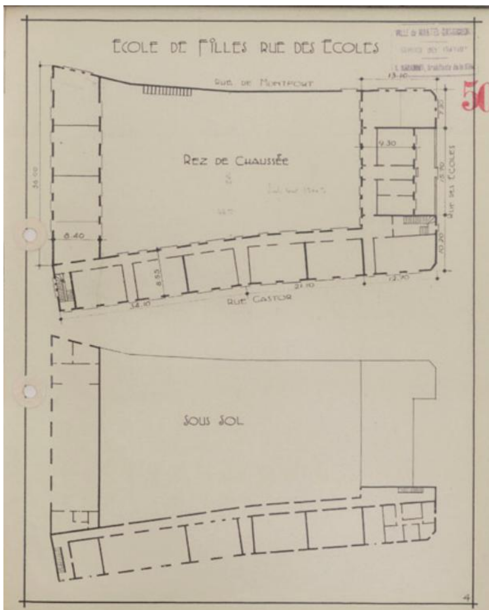
Plan du rez-de-chaussée et du sous-sol vers 1940. AM. Mantes-la-Jolie, 1 M 1.
