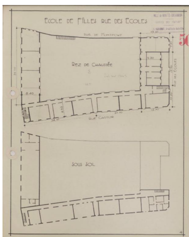
Plan du rez-de-chaussée et du sous-sol vers 1940. AM. Mantes-la-Jolie, 1 M 1. IVR11_20177800496NUC4A
