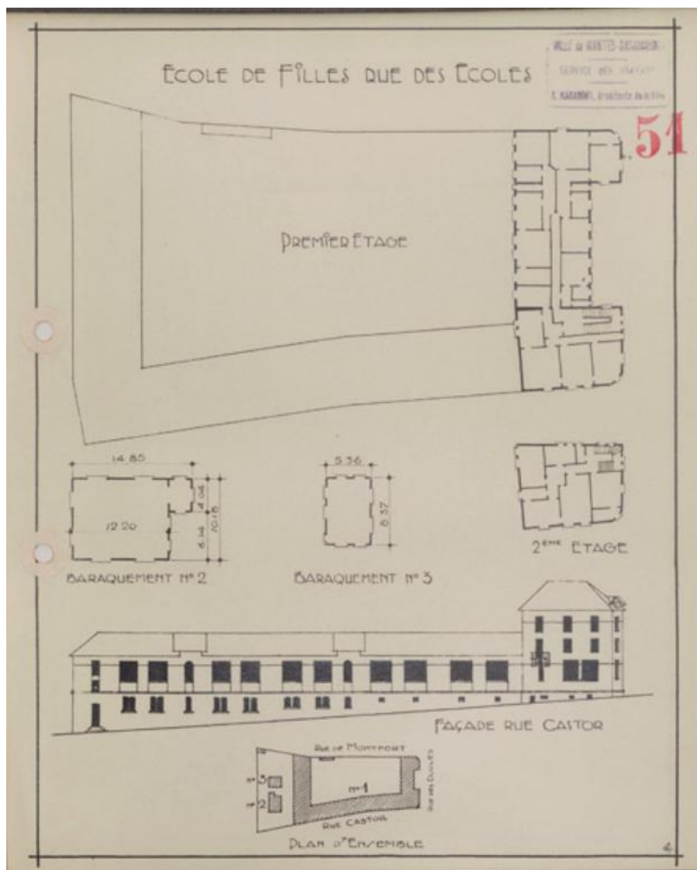
Plan et élévation de l'école vers 1940. AM. Mantes-la-Jolie, 1 M 1.
