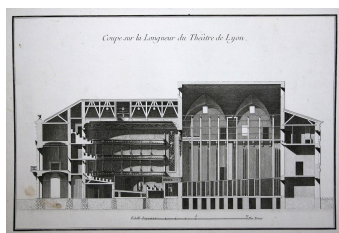
Coupe longitudinale du théâtre de Lyon, archives privées.
