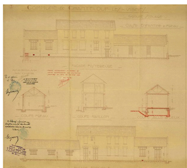
Projet d'agrandissement par Fourret : élévations des bâtiments de l'école enfantine. Dessin. (AD Yvelines, 2/050/1).
