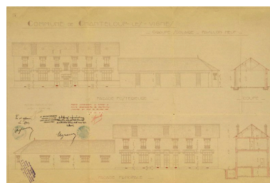
Projet d'agrandissement par Fourret : élévation des bâtiments nouveaux. Dessin. (AD Yvelines, 2/050/1).
