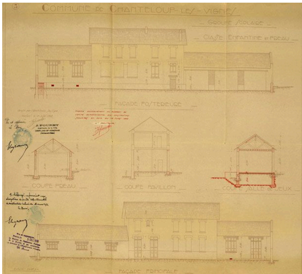
Projet d'agrandissement par Fouret : élévations des bâtiments de l'école enfantine. Dessin. (AD Yvelines, 2/050/1).
