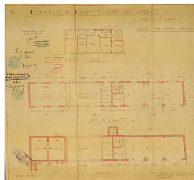
Projet d'agrandissement par Fourret : plan des bâtiments de l'école enfantine. Dessin. (AD Yvelines, 2/050/1).
