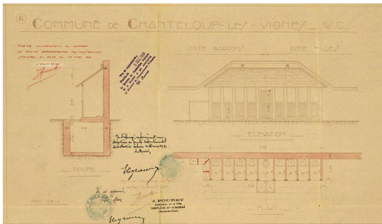
Projet d'agrandissement par Fouret : plan et élévation des WC. Dessin. (AD Yvelines, 2/050/1).
