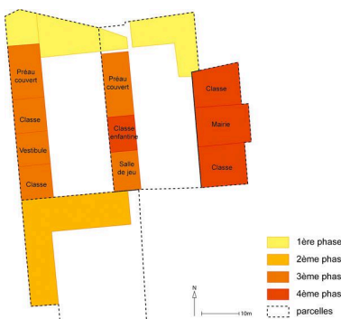
Les différentes étapes de construction. Dessin. (AD Yvelines, 2/050/1).
