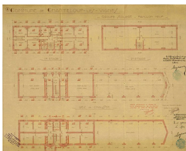
Projet d'agrandissement par Fourret : plans des bâtiments nouveaux. Dessin. (AD Yvelines, 2/050/1).
