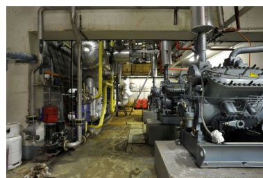
Vue des locaux techniques pour la fabrication de la glace : détail des machines Phot. Laurent Kruszyk IVR11_20129500268NUC4A
