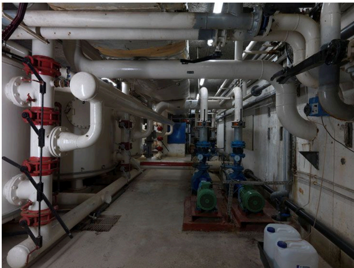
Piscine : détail d'un espace technique en sous-sol, la salle des machines.
