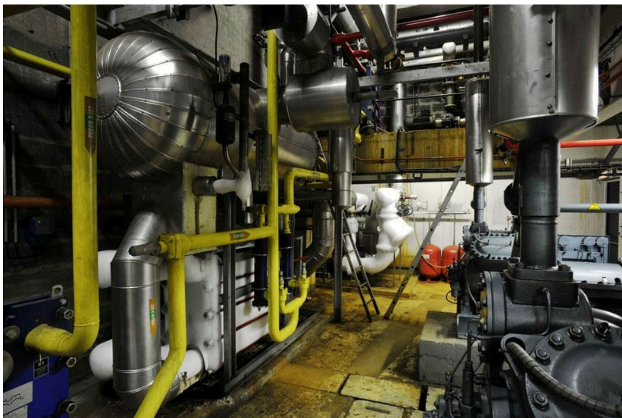
Vue des locaux techniques pour la fabrication de la glace : détail des machines
