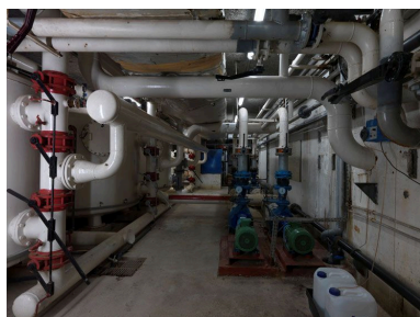
Piscine : détail d'un espace technique en sous-sol, la salle des machines. Phot. Laurent Kruszyk IVR11_20129500344NUC4A
