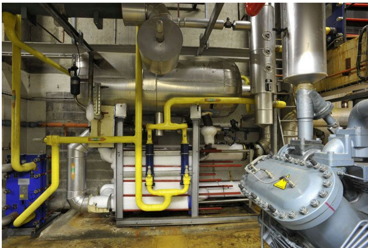
Vue des locaux techniques pour la fabrication de la glace : détail
