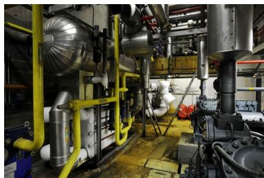
Vue des locaux techniques pour la fabrication de la glace : détail des machines Phot. Laurent Kruszyk IVR11_20129500269NUC4A
