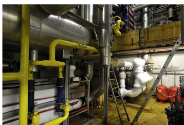
Vue des locaux techniques pour la fabrication de la glace : détail des machines Phot. Laurent Kruszyk IVR11_20129500267NUC4A
