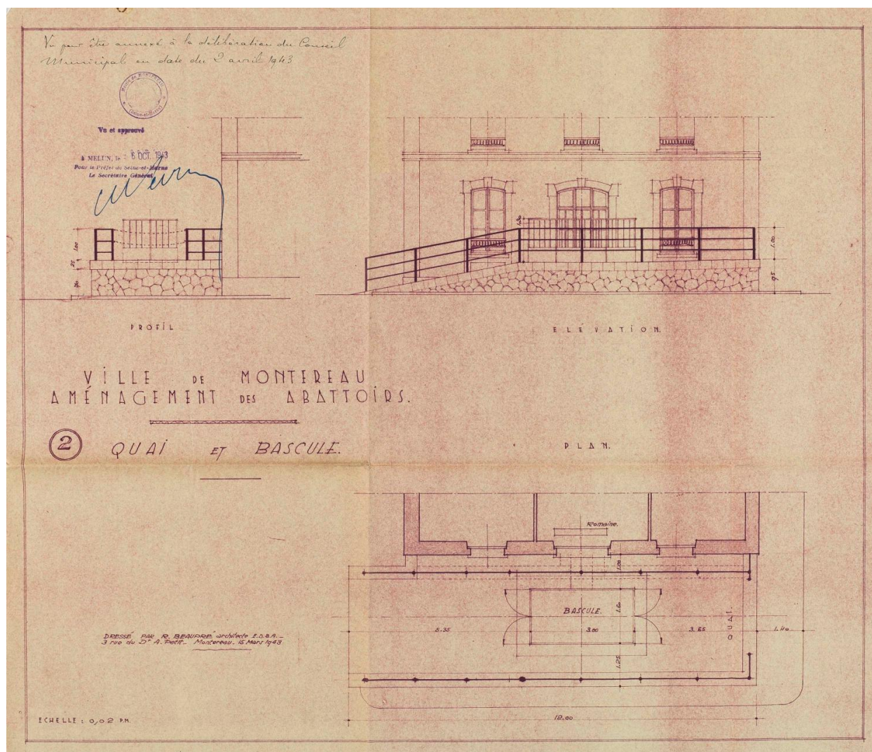
Plan d'aménagement des abattoirs, 1943.
