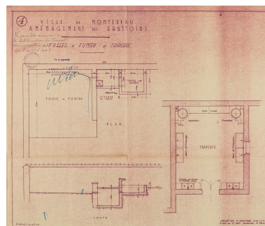
Plan d'aménagement des abattoirs, 1943. Repro. Yvan Bourhis, Autr. René Beaupré IVR11_20237700001NUC4A
