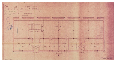
Plan d'aménagement des abattoirs, 1943. Repro. Yvan Bourhis, Autr. René Beaupré IVR11_20237700002NUC4A
