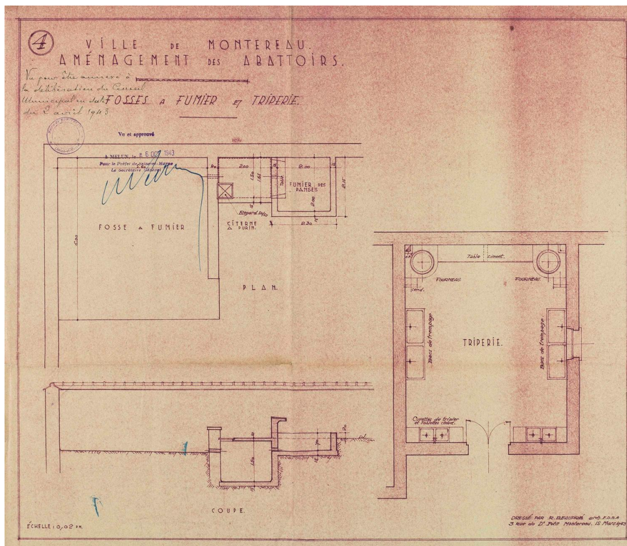
Plan d'aménagement des abattoirs, 1943.
