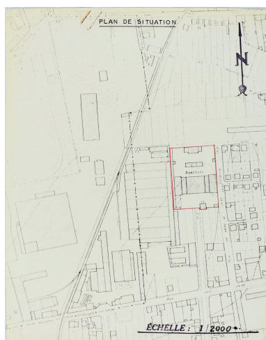
Plan de situation des abattoirs, 1960. (réf. Département Seine-et-Marne : IVD77_2014_77_00138_NUCA) Repro. Yvan Bourhis IVR11_20197700465NUC4A
