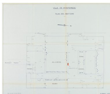
Plan des abattoirs, 1960. (réf. Département Seine-et-Marne : IVD77_2014_77_00139_NUCA) Repro. Yvan Bourhis IVR11_20197700466NUC4A
