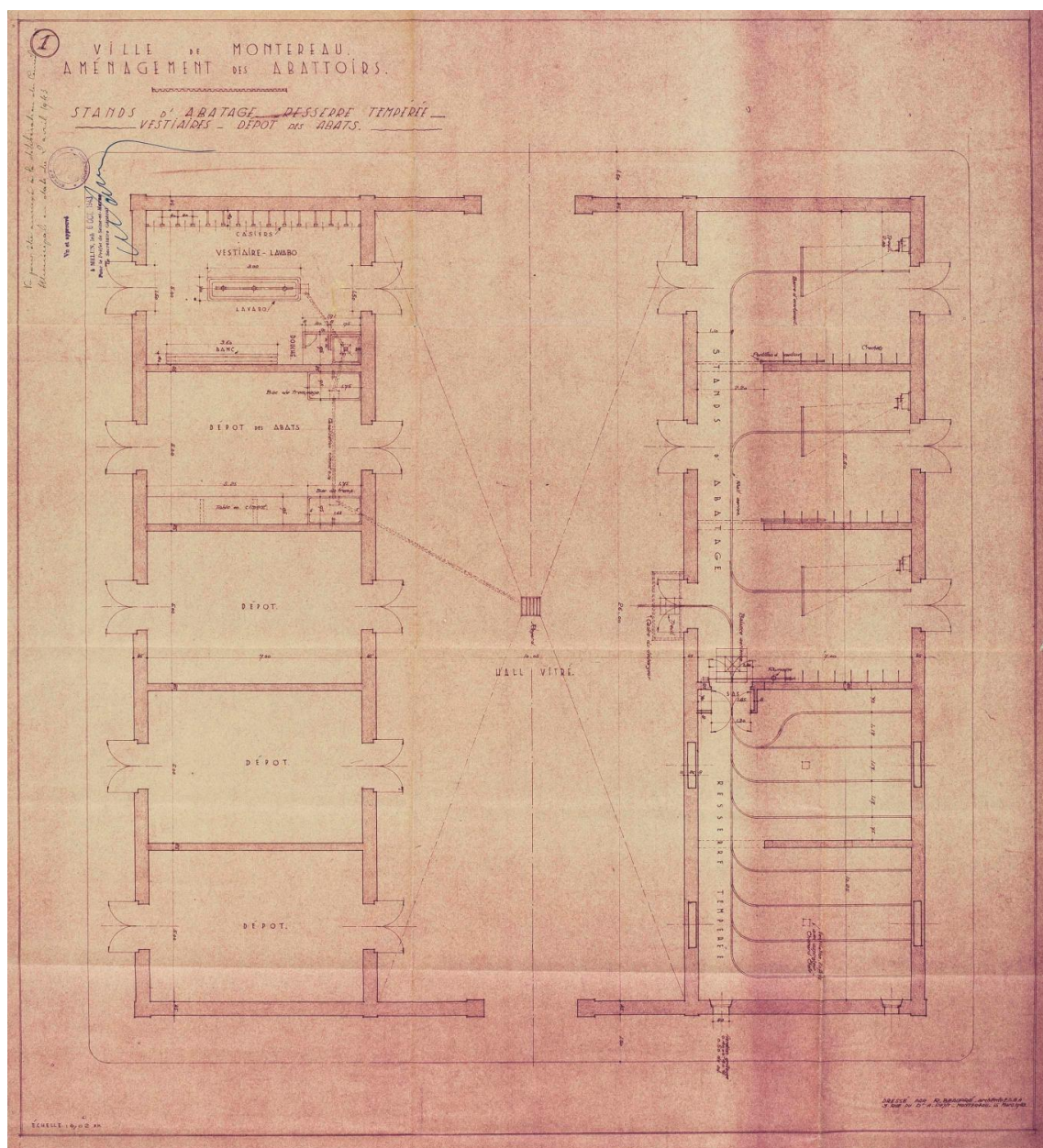
Plan d'aménagement des abattoirs, 1943.
