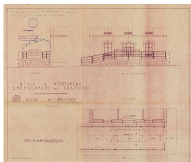
Plan d'aménagement des abattoirs, 1943. Repro. Yvan Bourhis, Autr. René Beaupré IVR11_20237700003NUC4A
