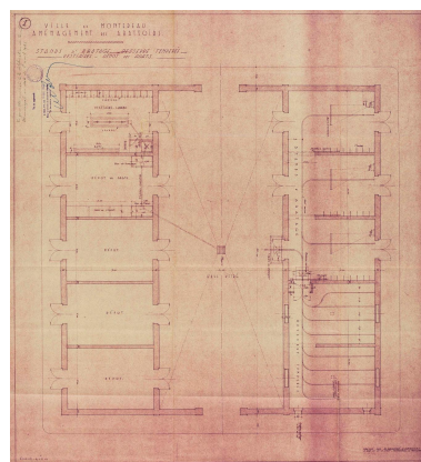
Plan d'aménagement des abattoirs, 1943. Repro. Yvan Bourhis, Autr. René Beaupré IVR11_20237700004NUC4A
