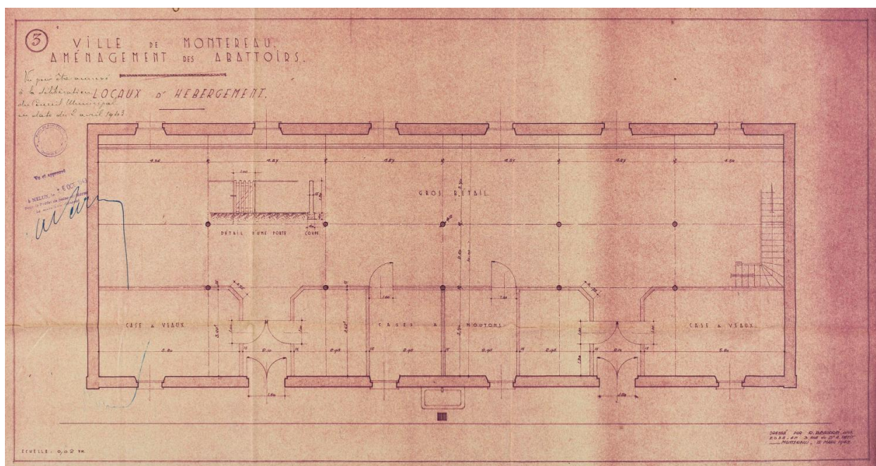
Plan d'aménagement des abattoirs, 1943.
