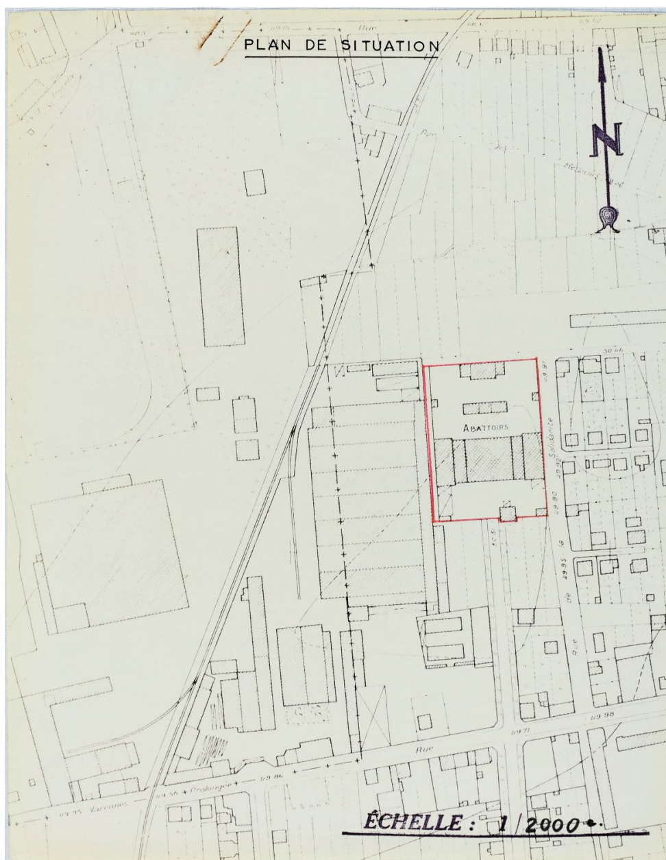
Plan de situation des abattoirs, 1960. (réf. Département Seine-et-Marne : IVD77_2014_77_00138_NUCA)
