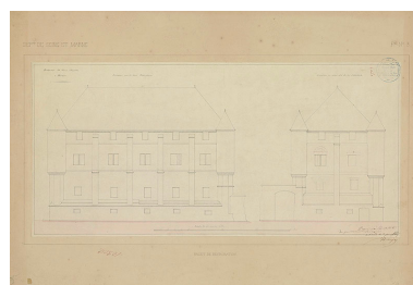
Projet de restauration, par Danjoy (1845) : élévations sur la rue Notre-Dame (mur gouttereau est) et vers la cathédrale (mur pignon sud). Papier aquarellé, 3 juin 1845. (Médiathèque de l'architecture et du patrimoine. 0082/077/2019.) Phot. Réunion des musées nationaux, Autr. Danjoy (architecte) IVR11_20127700996NUC2A
