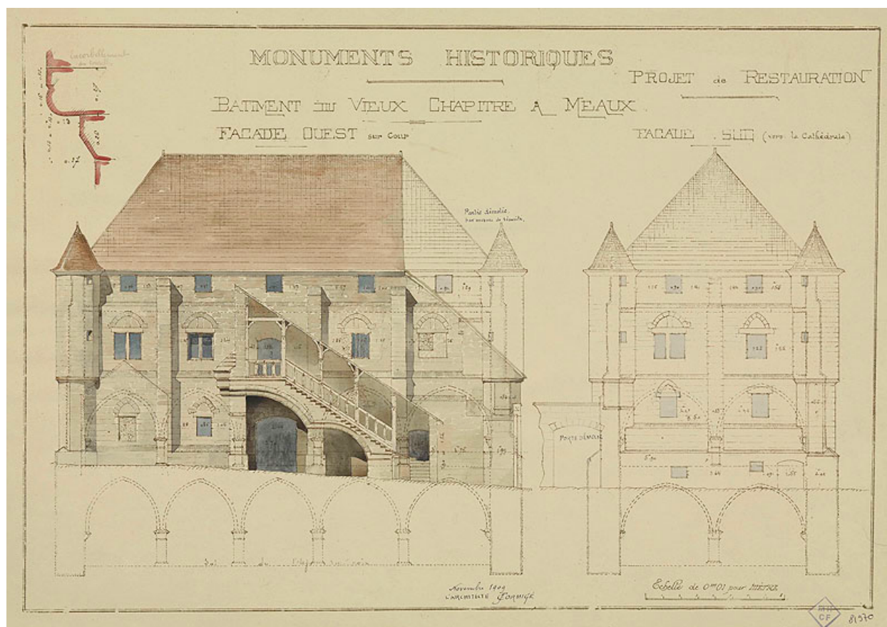
Projet de restauration, par Formigé (1909) : élévations ouest et sud. Papier aquarellé, novembre 1909. (Médiathèque de l'architecture et du patrimoine. 0082/077/2019, document n°081970.)
