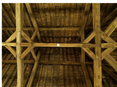
La charpente : vue de deux fermes. Phot. Stéphane Asseline IVR11_20087701001NUC4A
