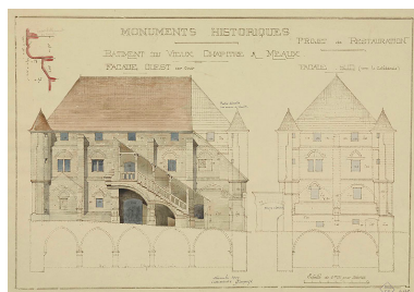
Projet de restauration, par Formigé (1909) : élévations ouest et sud. Papier aquarellé, novembre 1909. (Médiathèque de l'architecture et du patrimoine. 0082/077/2019, document n°081970.) Phot. Réunion des musées nationaux, Autr. Formigé (architecte)
