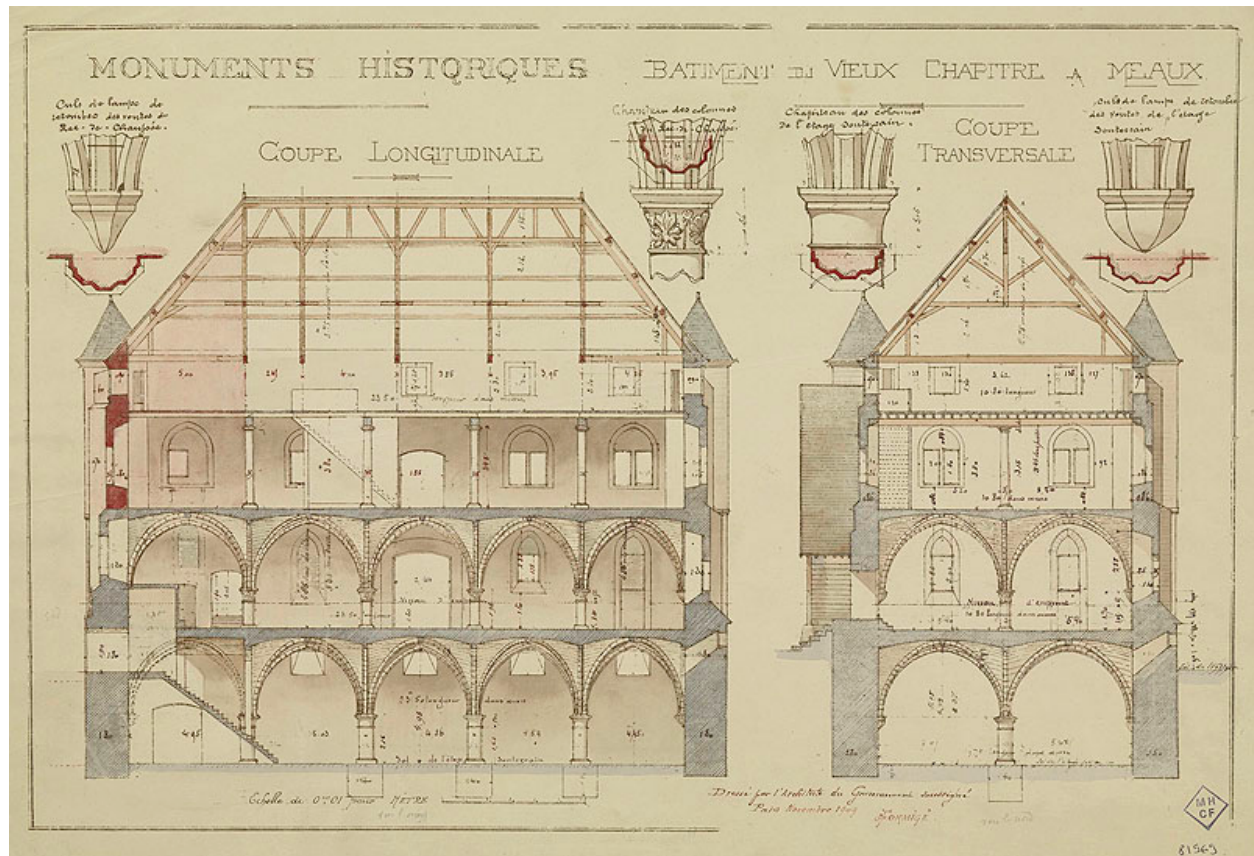
Projet de restauration, par Formigé (1909) : coupes longitudinale et transversale. Papier aquarellé, novembre 1909. (Médiathèque de l'architecture et du patrimoine. 0082/077/2019, document n°081969.)
