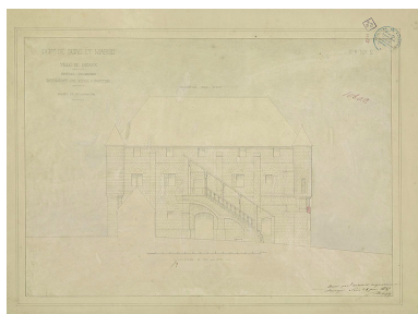
Projet de restauration, par Danjoy (1845) : élévation ouest. Papier aquarellé, 3 juin 1845. (Médiathèque de l'architecture et du patrimoine. 0082/077/2019.) Phot. Réunion des musées nationaux, Autr. Danjoy (architecte)
