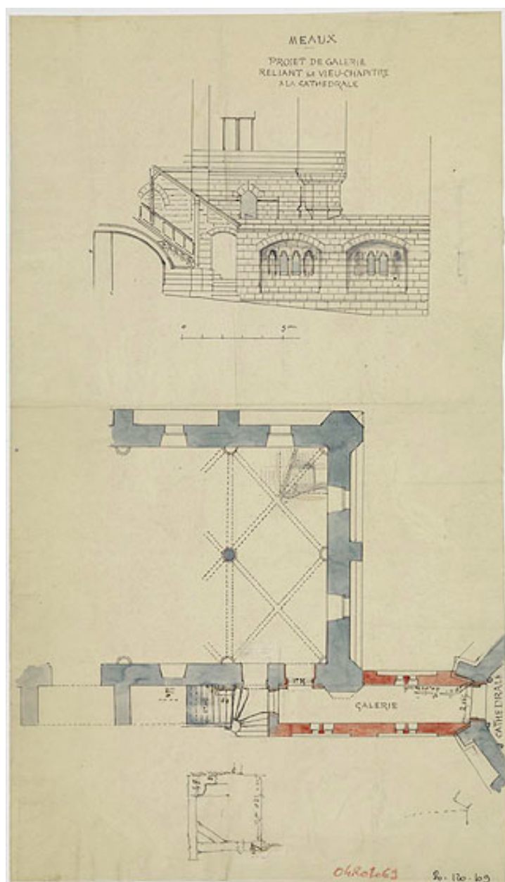
Projet (non réalisé) de galerie reliant le Vieux-Chapitre à la cathédrale. (Médiathèque de l'architecture et du patrimoine. 0080/120/1002, document n°109.)
