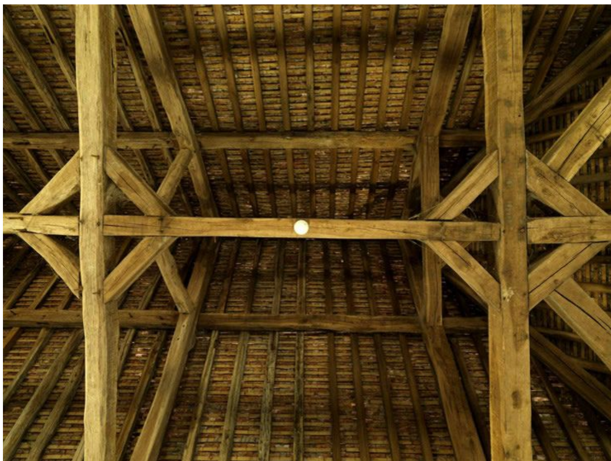
La charpente : vue de deux fermes.
