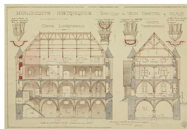
Projet de restauration, par Formigé (1909) : coupes longitudinale et transversale. Papier aquarellé, novembre 1909. (Médiathèque de l'architecture et du patrimoine. 0082/077/2019, document n°081969.) Phot. Réunion des musées nationaux, Autr. Formigé (architecte)
