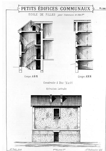
Coupe et élévation latérale. IVR11_20007800061X
