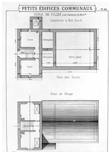
Plan des caves et de l'étage. IVR11_20007800062X
