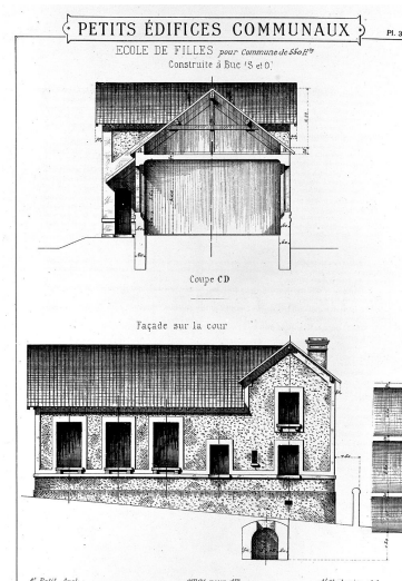
Coupe et élévation sur cour. IVR11_20007800063X
