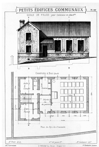
La façade sur rue et le plan du rez-de-chaussée. IVR11_20007800064X
