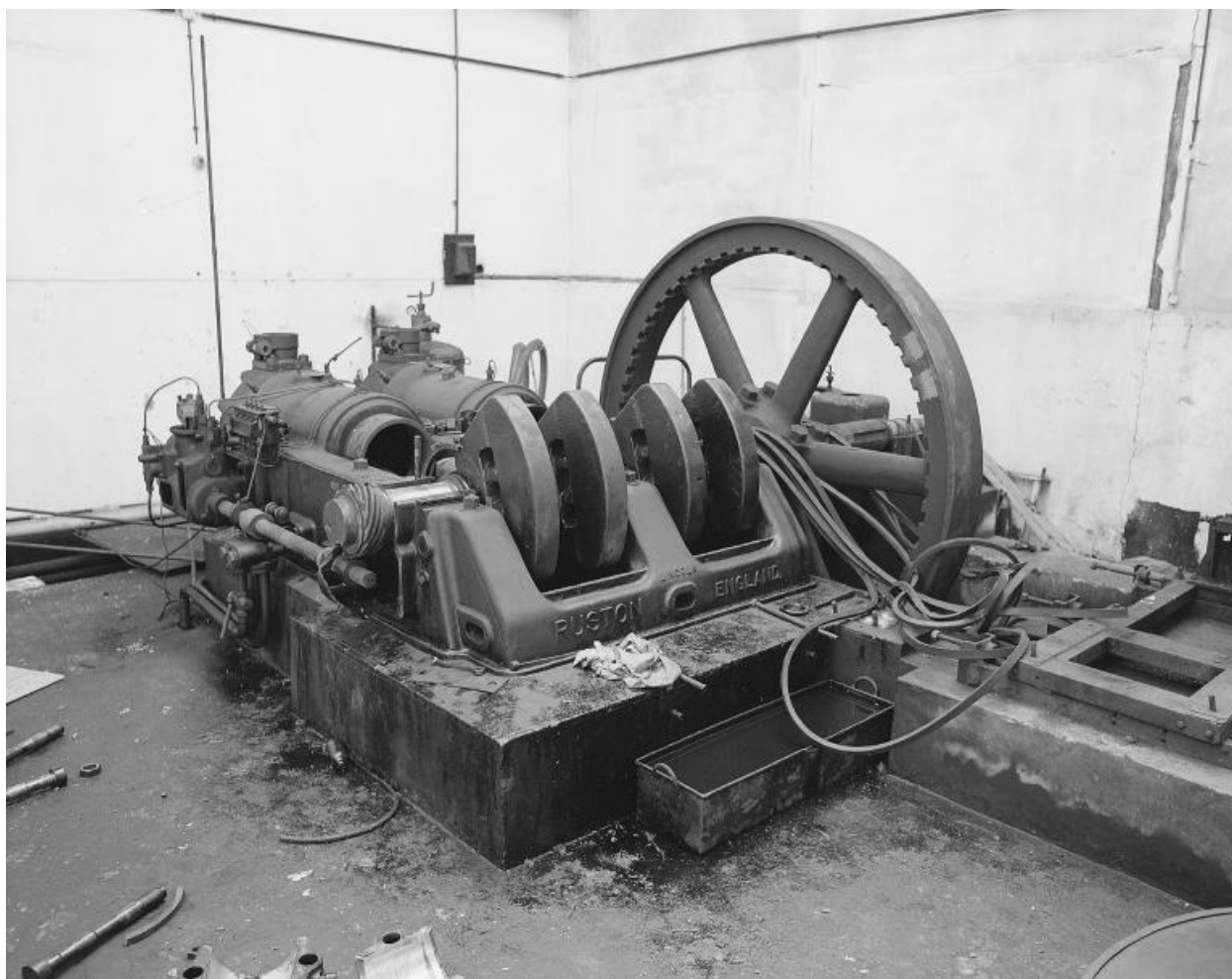
moteur Ruston des générateurs de la centrale électrique, vers 1988. Photographie. (AD Seine-Saint-Denis. A NB 118)
