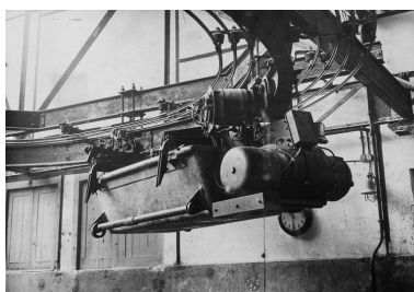
Chariot aérien, vers 1990. Photographie. (AD Seine-Saint-Denis. A NB 118) IVR11_20029300097NUC
