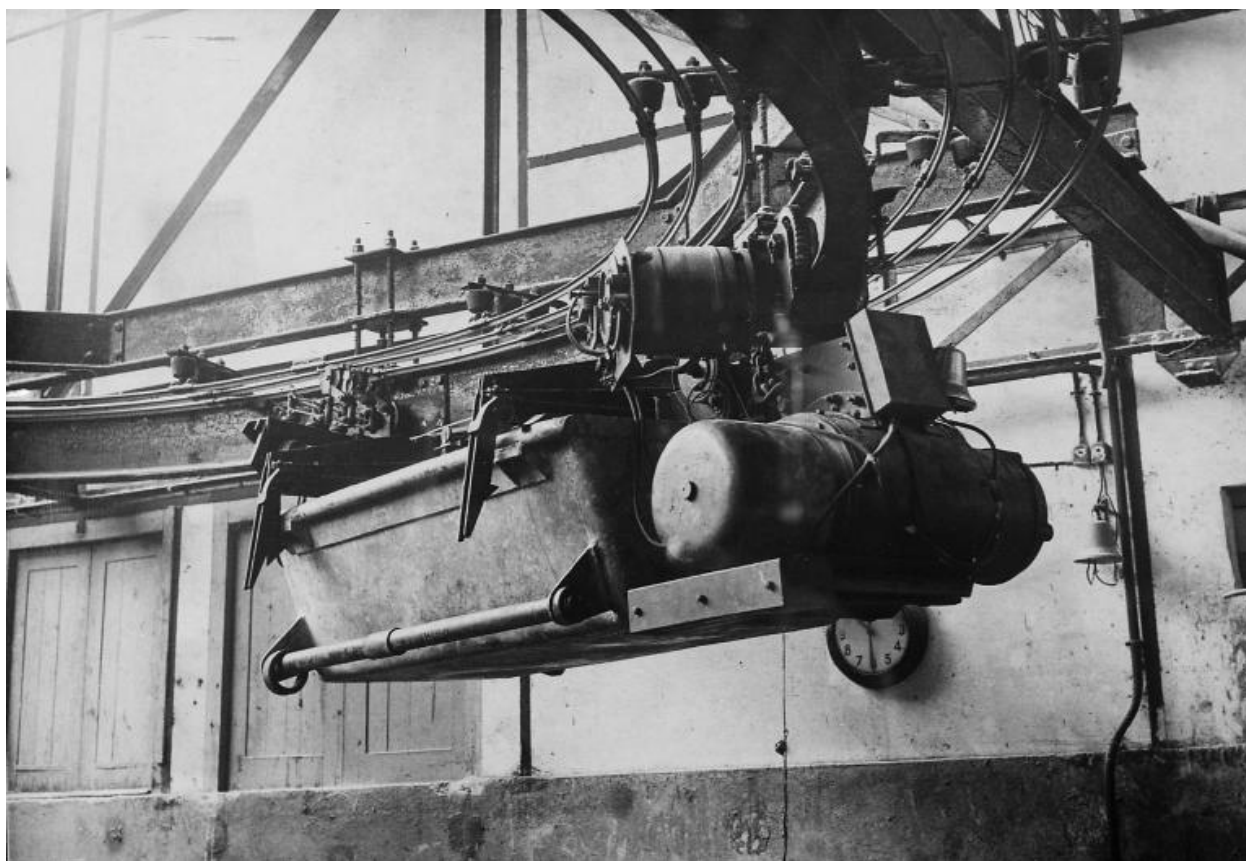
Chariot aérien, vers 1990. Photographie. (AD Seine-Saint-Denis. A NB 118)
