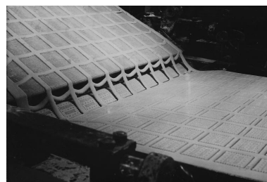
bande transporteuse de pâtes à biscuit, après découpe, vers 1960. Photographie. (AD Seine-Saint-Denis. A NB 118) IVR11_20029300101NUC
