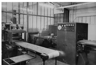
vue générale d'un atelier, vers 1960. Photographie. (AD Seine-Saint-Denis. A NB 118) IVR11_20029300099NUC
