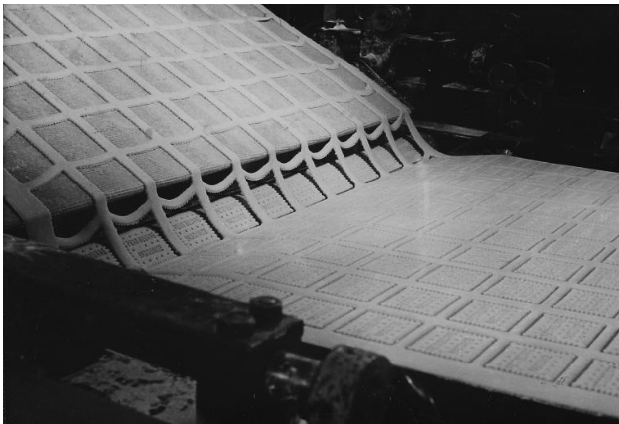
bande transporteuse de pâtes à biscuit, après découpe, vers 1960. Photographie. (AD Seine-Saint-Denis. A NB 118)
