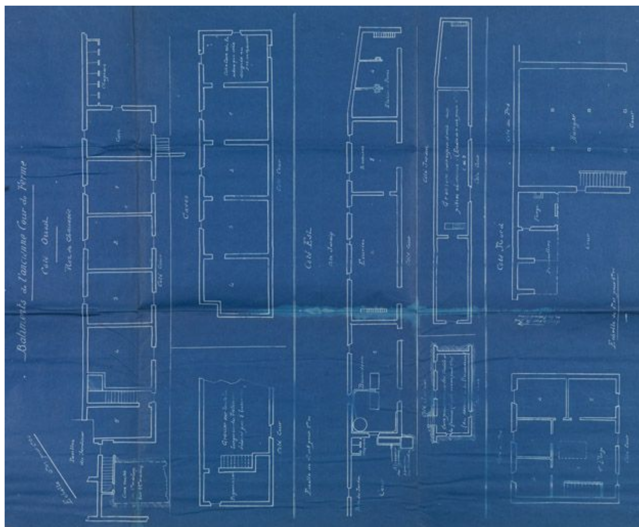
Plans des bâtiments de l'ancienne cour de ferme, côtés ouest, est et nord. (AD Essonne, 1 J 155)
