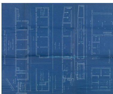
Plans des bâtiments de l'ancienne cour de ferme, côtés ouest, est et nord. (AD Essonne, 1 J 155) Autr. Paul (architecte) Simon IVR11_20089100412NUC4A
